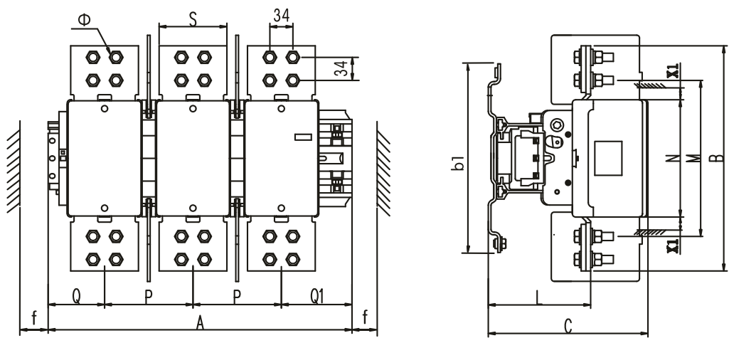
CJX2sF-1450、1700、2100 外形
