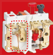
片簧式动触头
