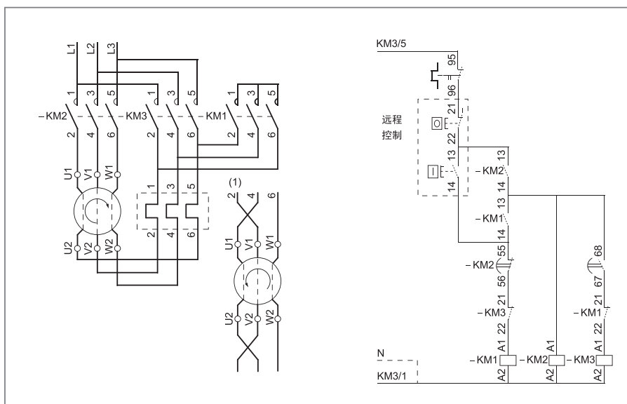
■ 星-三角启动器接线图
