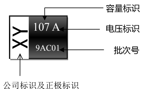
图 2 产品标识图
