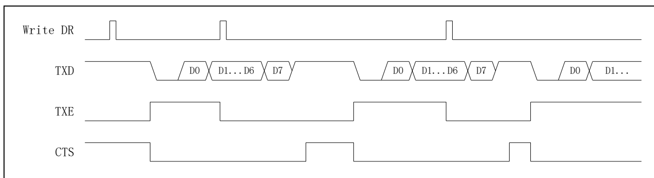
图 17-9 CTS 硬件流控信号
