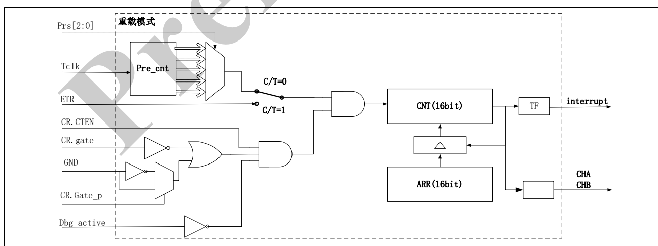
图 13-3 重载计数框图
