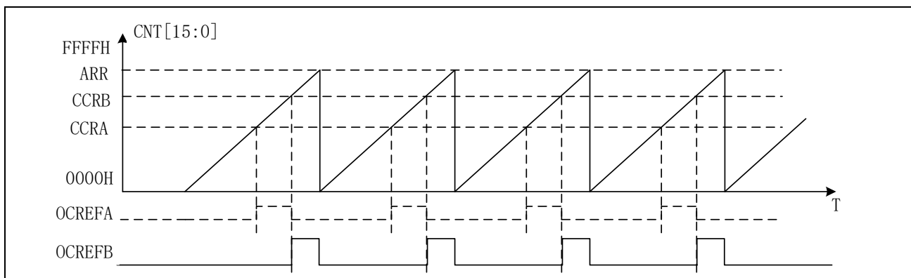
图 13-34 锯齿波计数双点比较 OCREF 输出 (OCM x =111)
