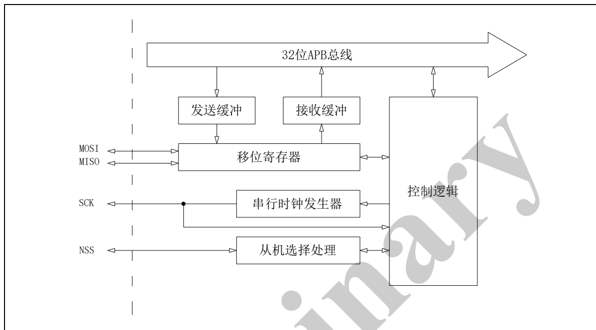
图 18-1 SPI 框图
