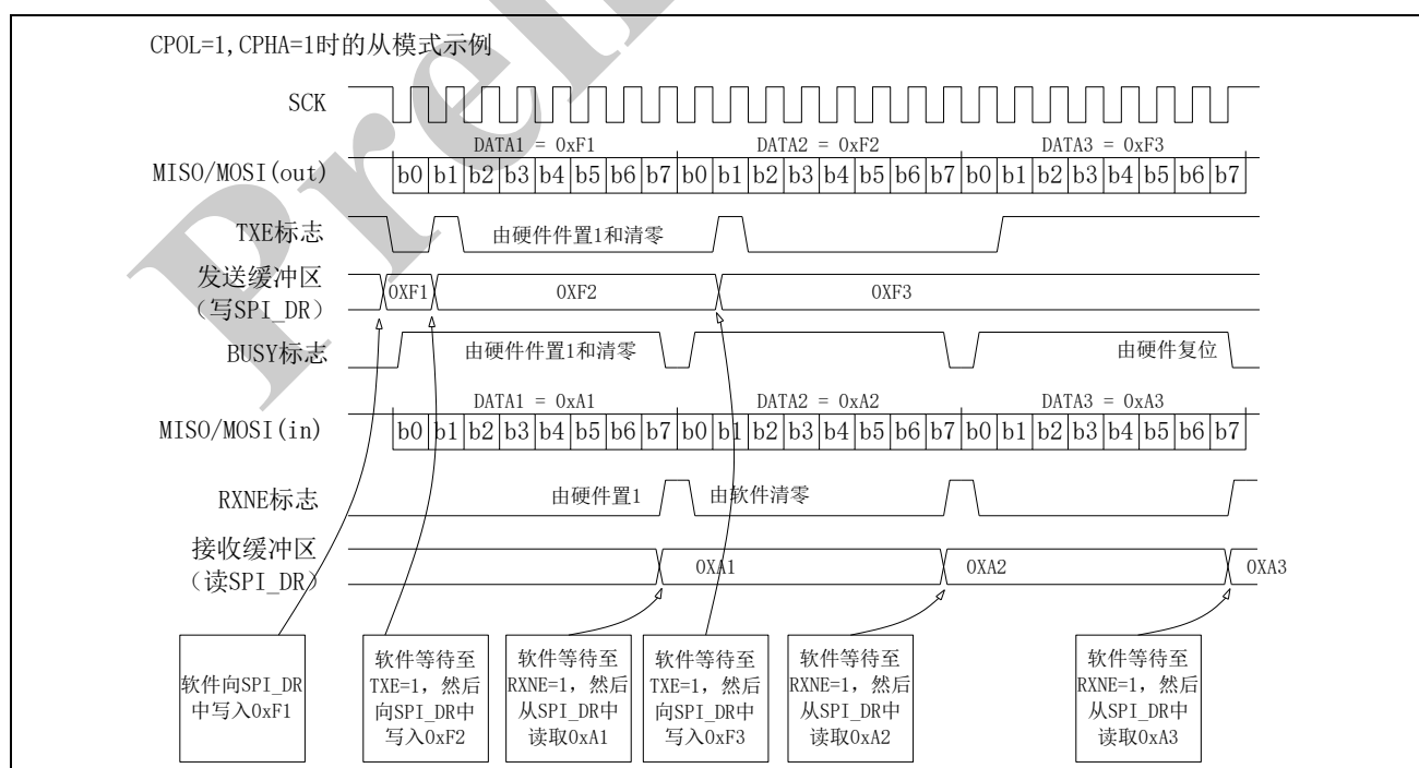
图 18-9 SPI 从机模式一般标志位说明图
