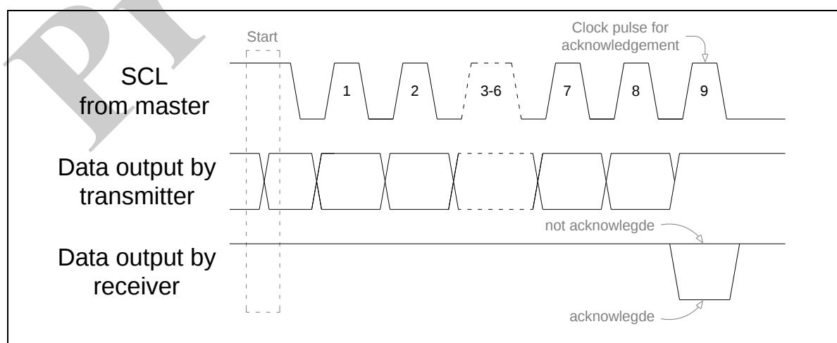
图 19-4 I2C 总线上应答信号
