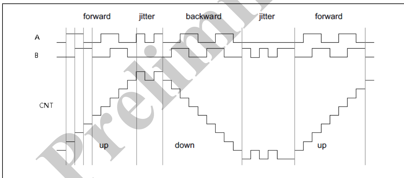
图 13-54 编码计数
