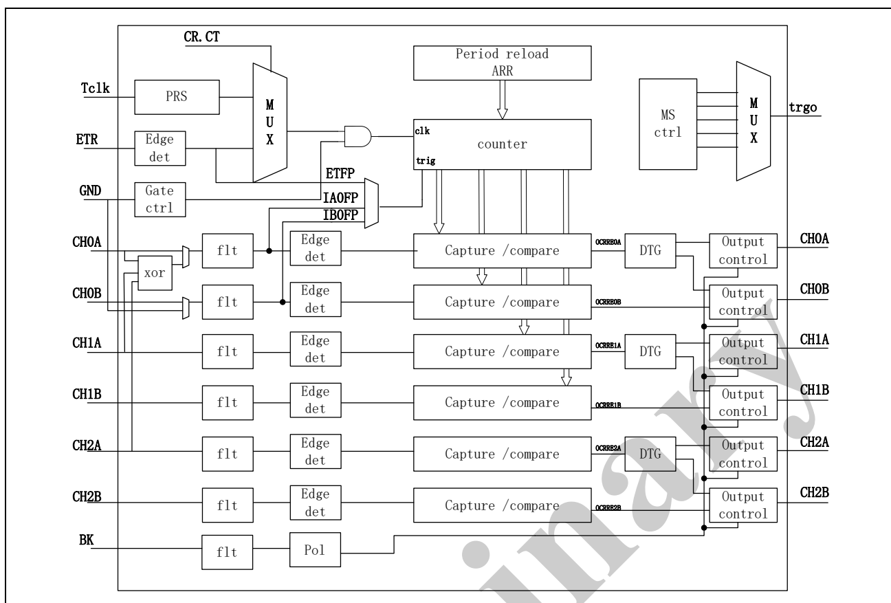
图 13-1 ATIM3 框图
