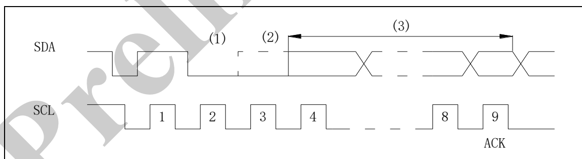
图 19-5 I2C 总线上的仲裁
