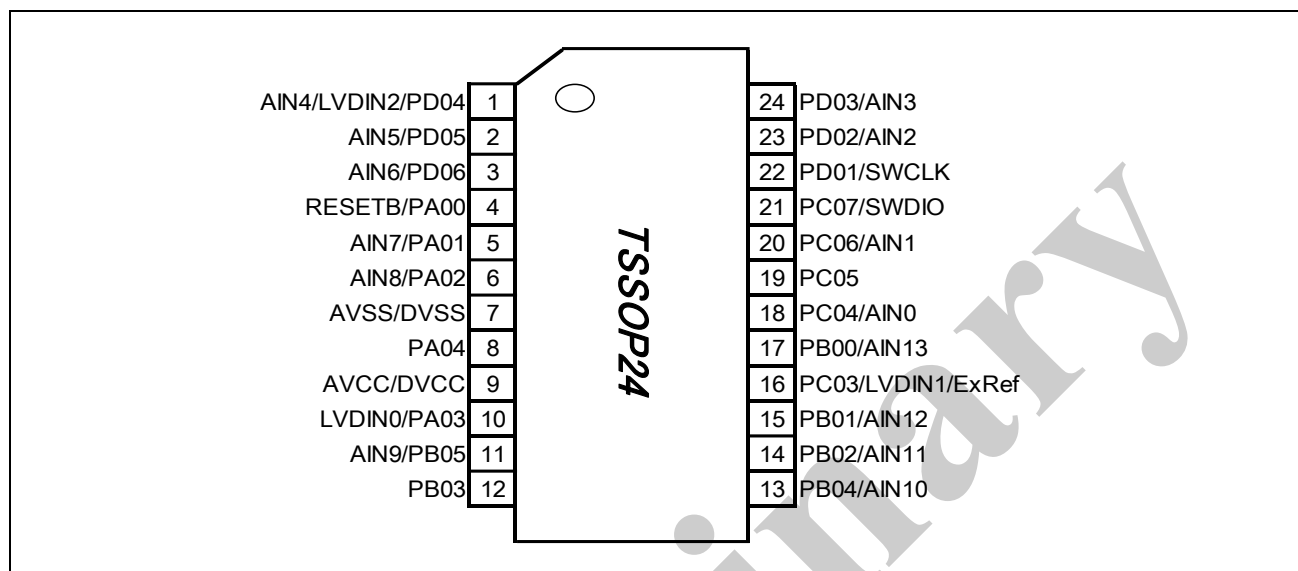
HC32F002D4PB-TSSOP24
