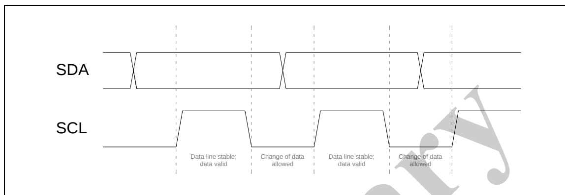
图 19-3 I2C 总线上传输
