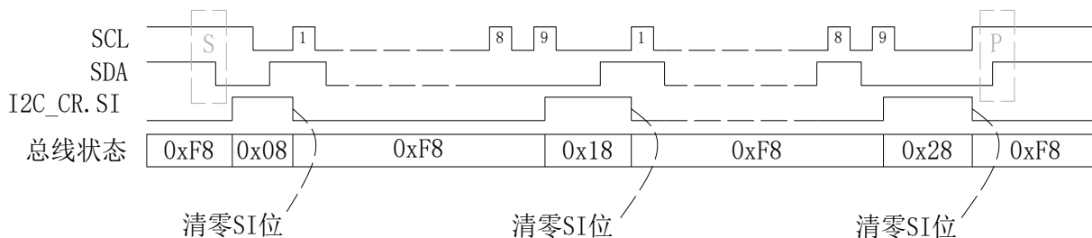
图 19-7 主发送模式数据同步图
