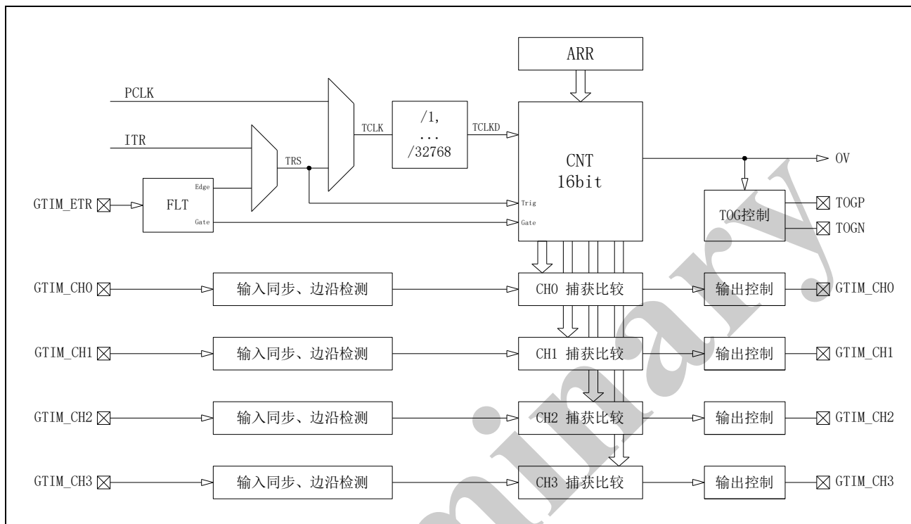
图 12-1 GTIM 框图
