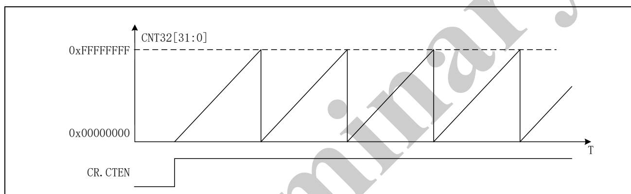
图 13-5 32位自由计数波形
