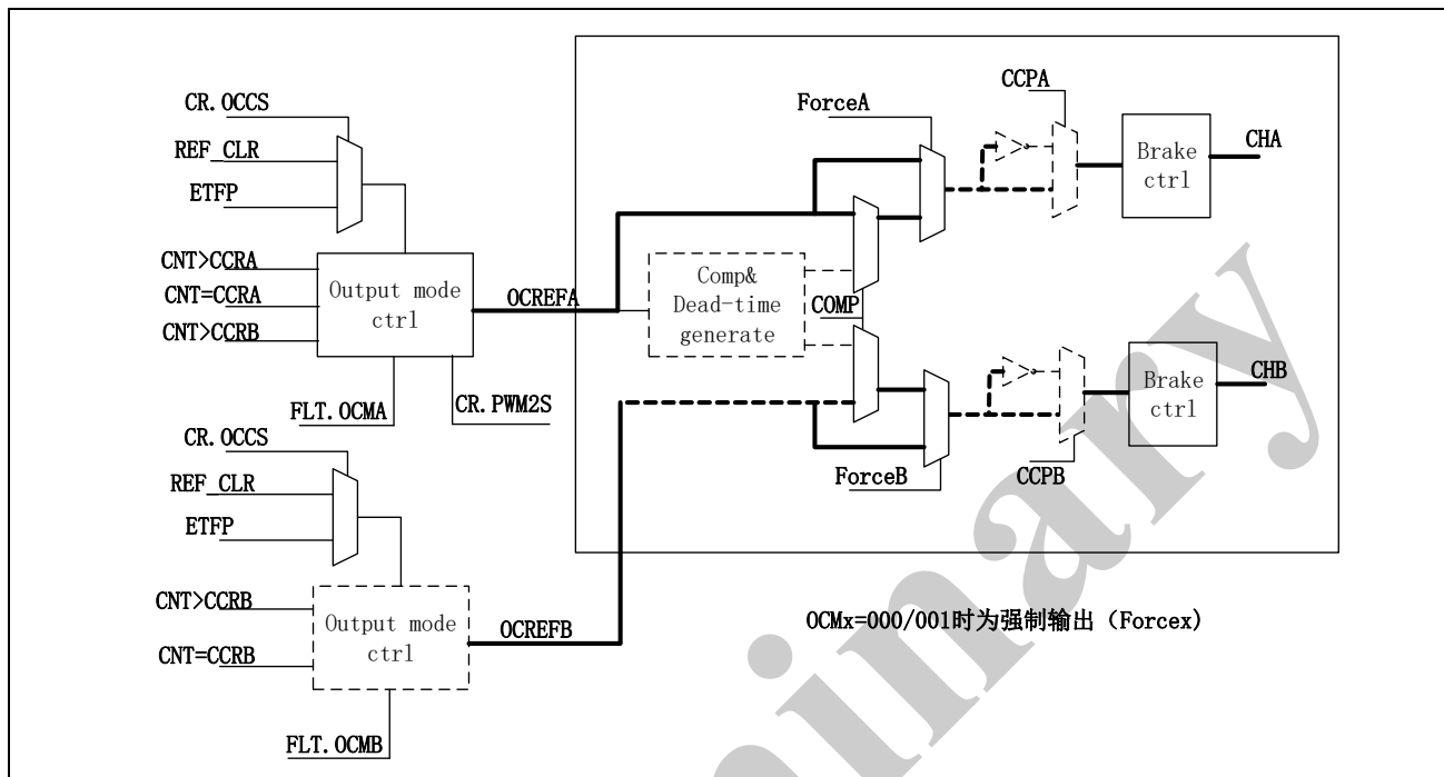
图 13-36 独立 PWM 输出框图
