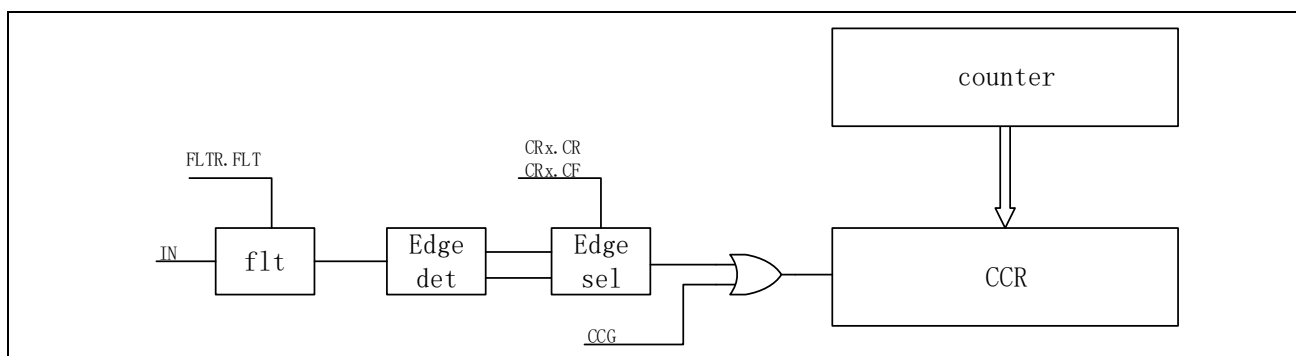
图 13-47 捕获功能框图
