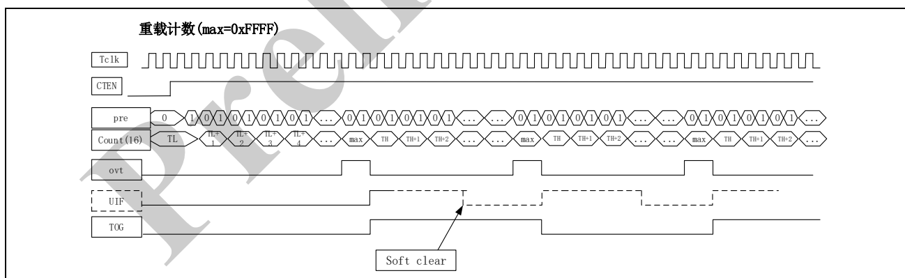
图 13-7 重载计数时序图（预分频设置为2）
