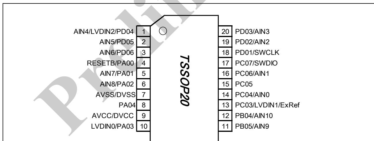
HC32F002C4PB-TSSOP20
