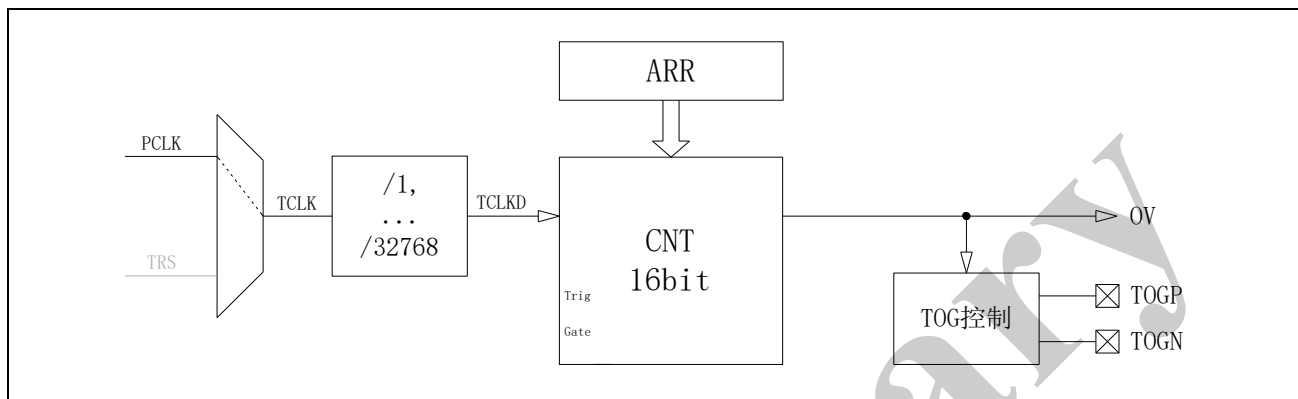
图 12-3 定时模式框图
