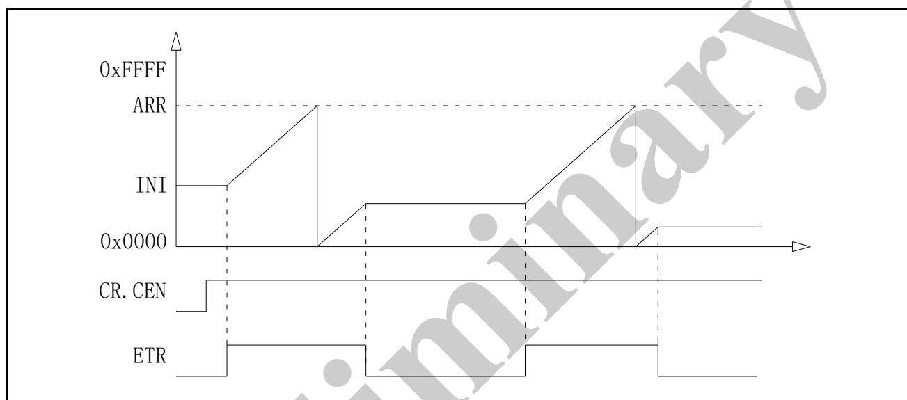
图 11-8 门控模式计数示意图
