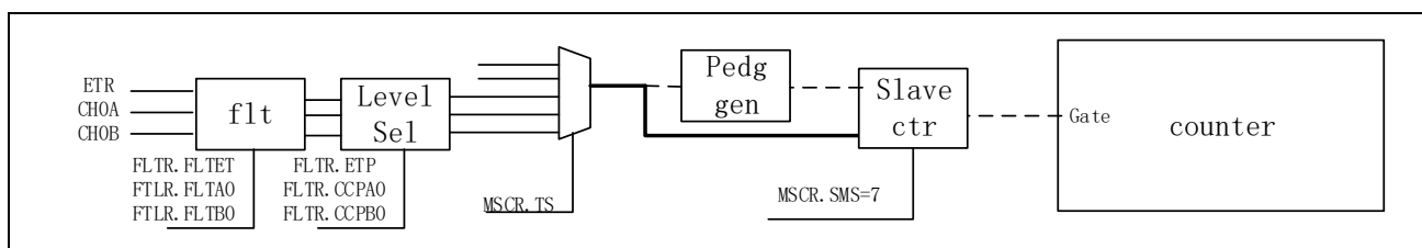
图 13-52 门控功能
