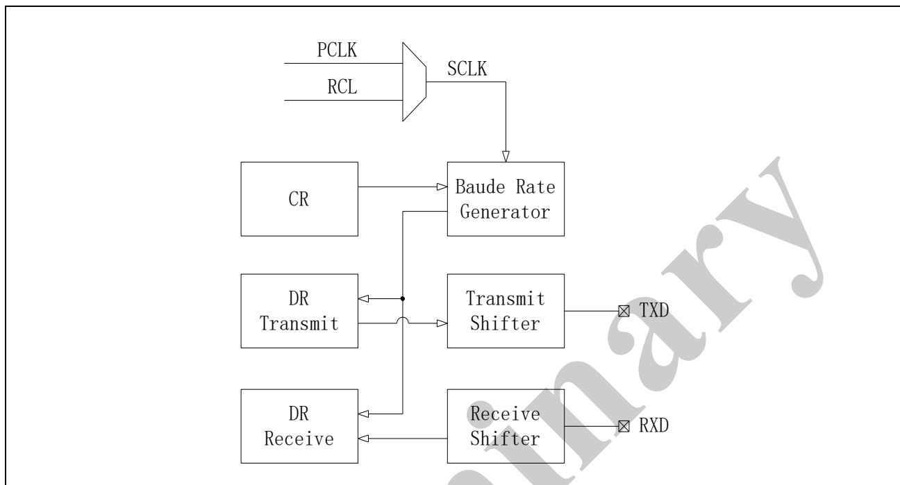
图 17-1 结构框图
