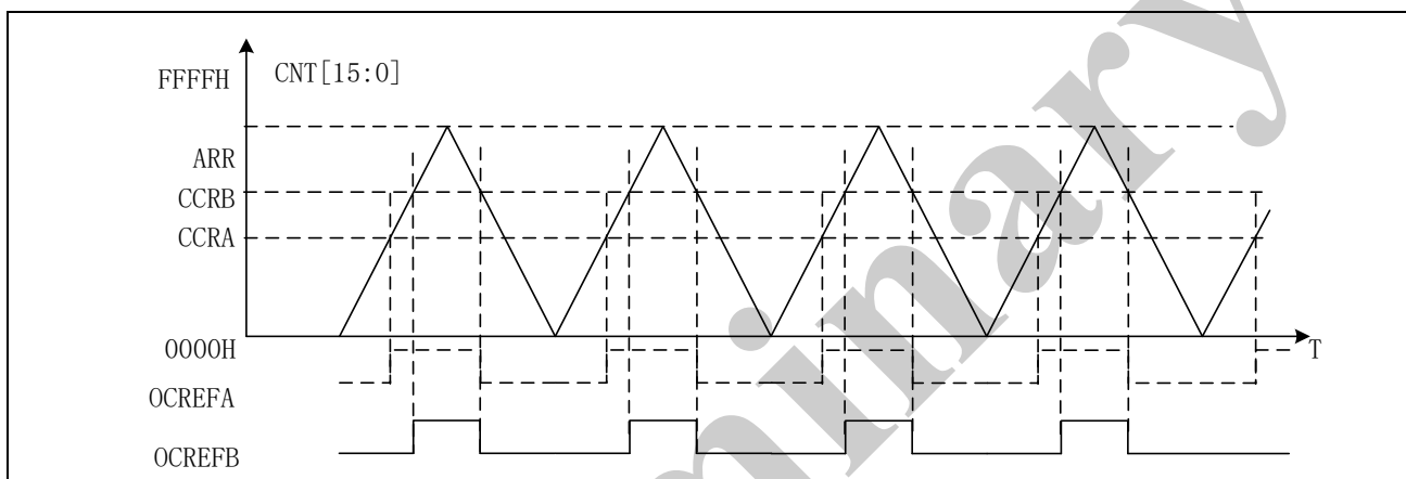
图 13-35 三角波计数双点比较 OCREF 输出 (OCM x =111)
