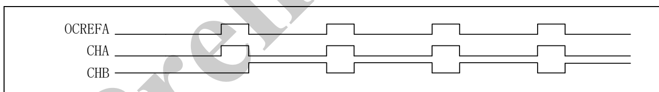
图 13-40 互补 PWM 输出波形图
