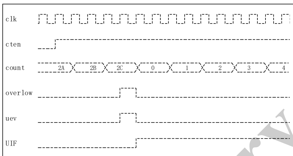
图 13-15 带预分频的上计数
