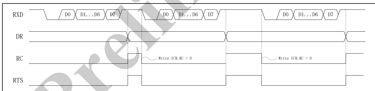
图 17-8 RTS 硬件流控信号
