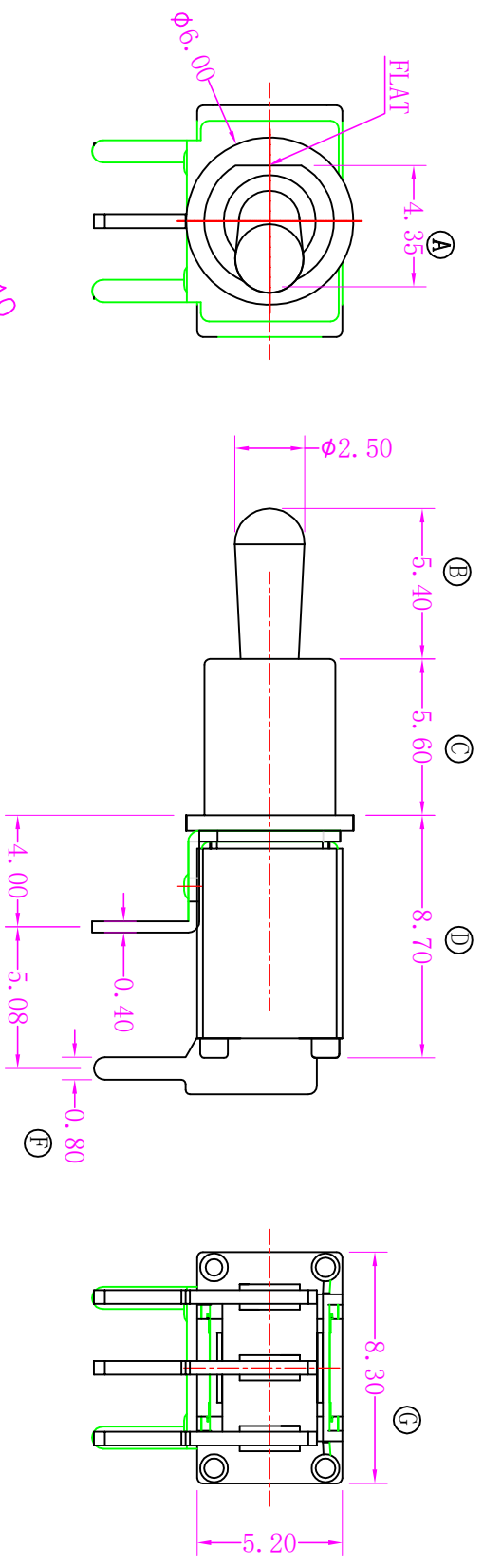
手柄位置及导通端子示意图
