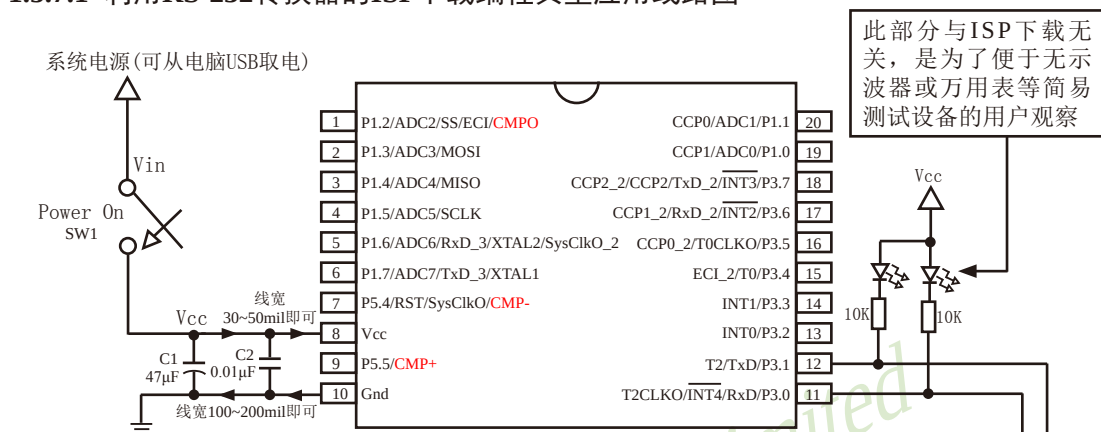
STC 单片机在线编程线路, STC RS-232 转换器
