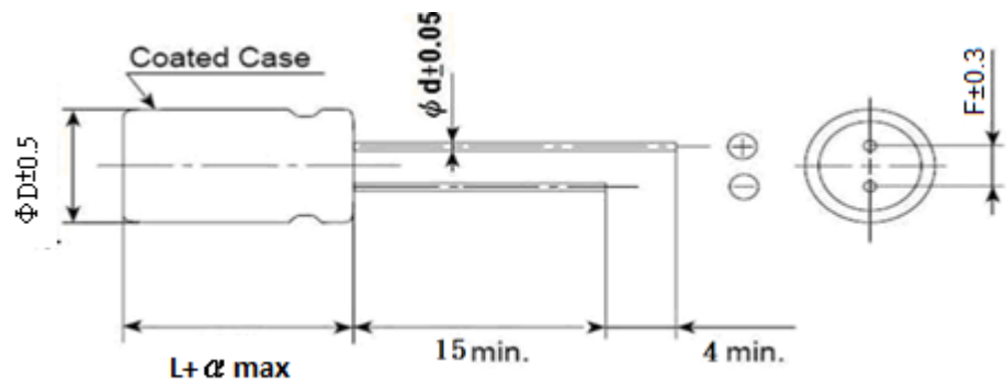
Fig. 2 Dimension
