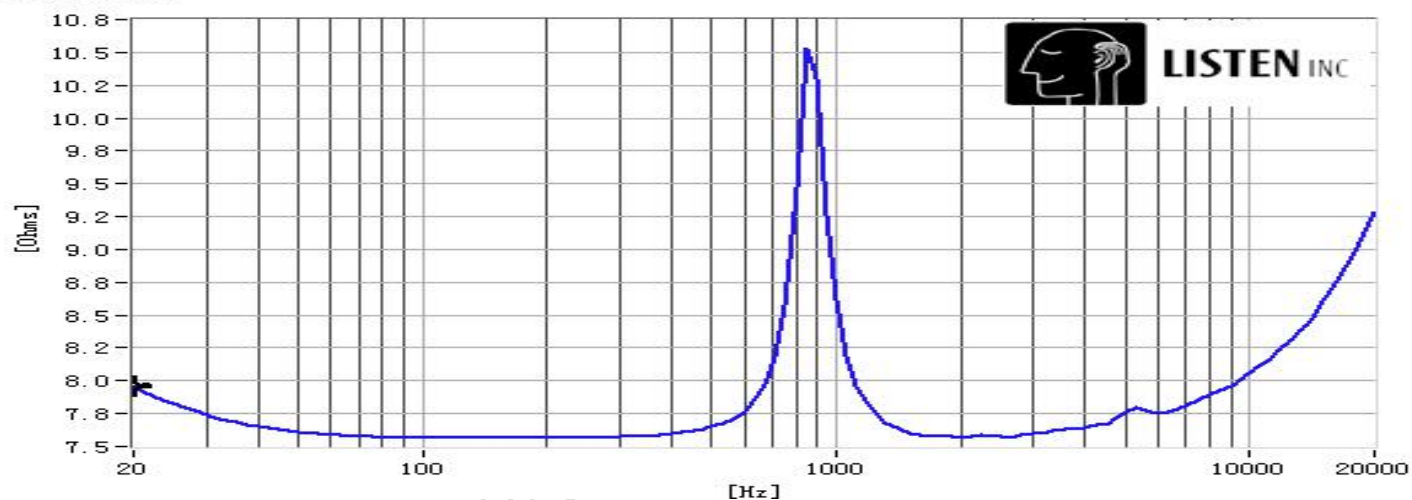
阻抗曲线
