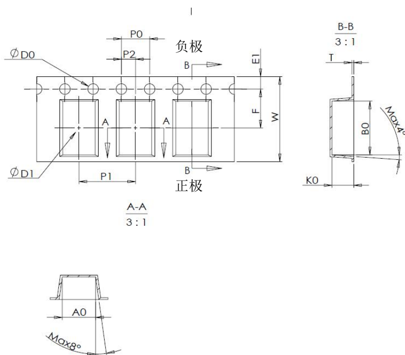
图 3 PX-Cap 包装带尺寸图
