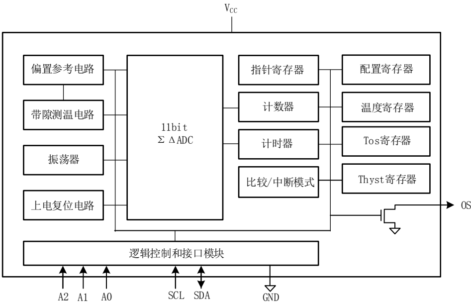
图 1. 芯片结构图
