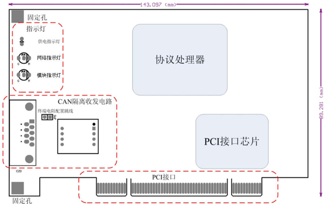
图 3.1 PCI-5010-D 结构框图
