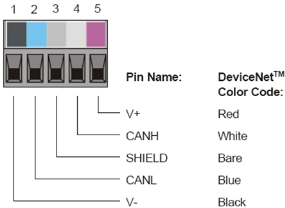
图 3.2 CAN Connect
