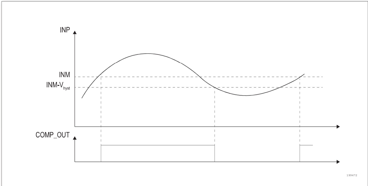
图29. 比较器的迟滞现象
