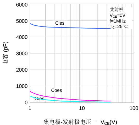
图8. 电容特性
