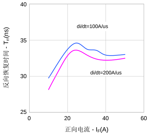
图 17. 反向恢复时间VS.正向电流
