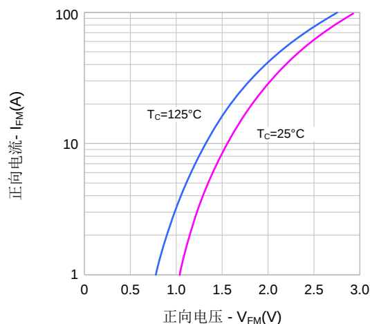
图16. 正向特性
