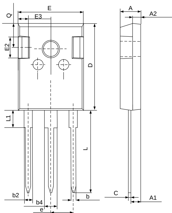
TO-247-3L
