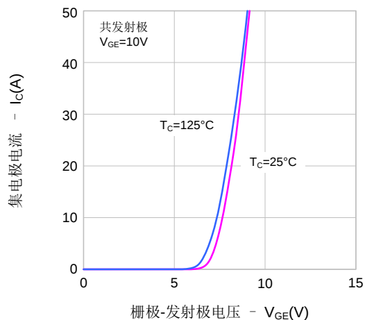
图4. 传输特性
