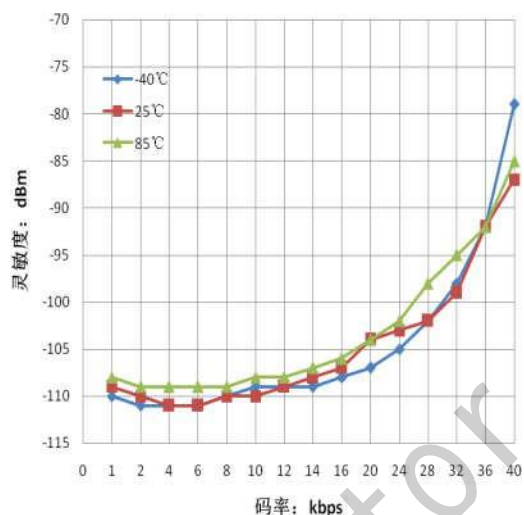
图8 315MHz 时，三温灵敏度随码率变化图
