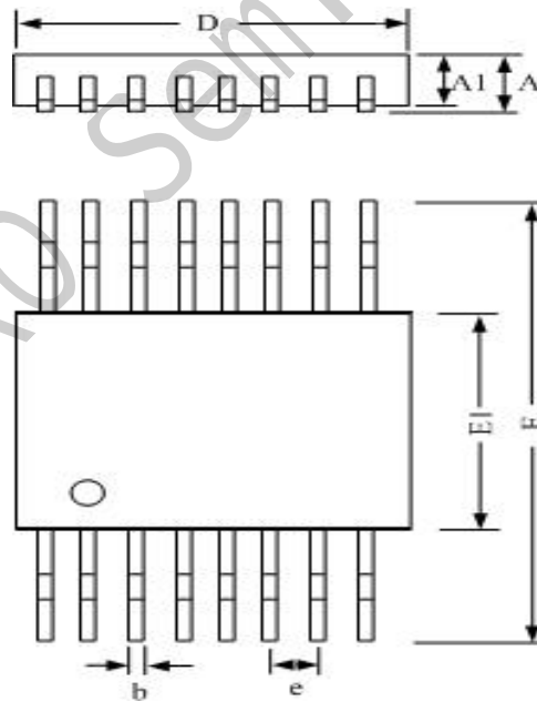
图 14 JSM500R型 封装外形图
