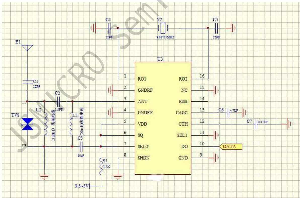
图 12 315MHz 工作模式原理图
