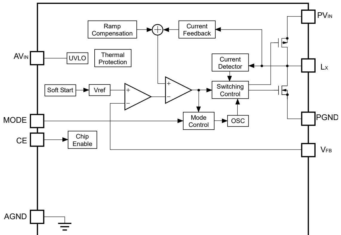
RP505K001C
