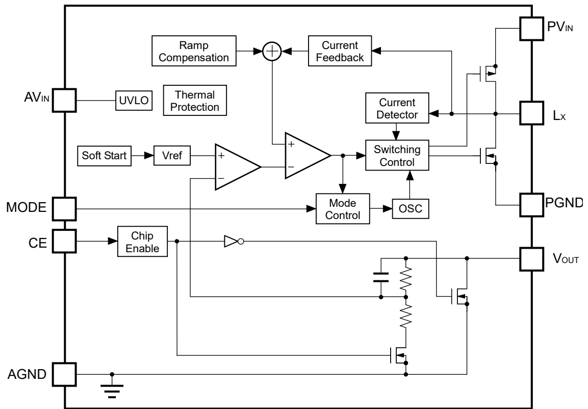
RP505K001C
