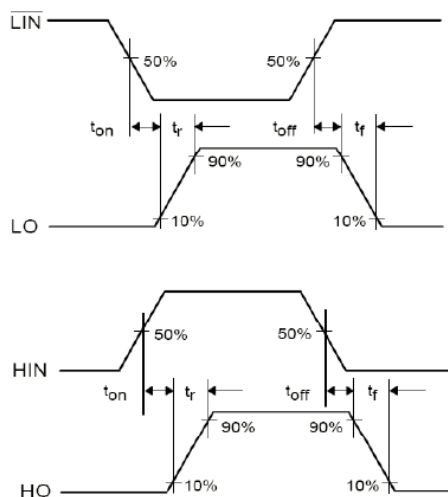
图 5-1 时序参数 t_{on}/t_{off}/t_f 定义
