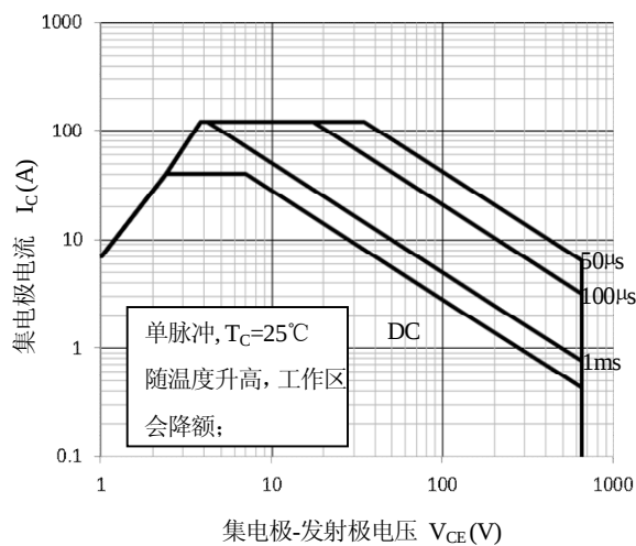
图 12. 安全工作区
