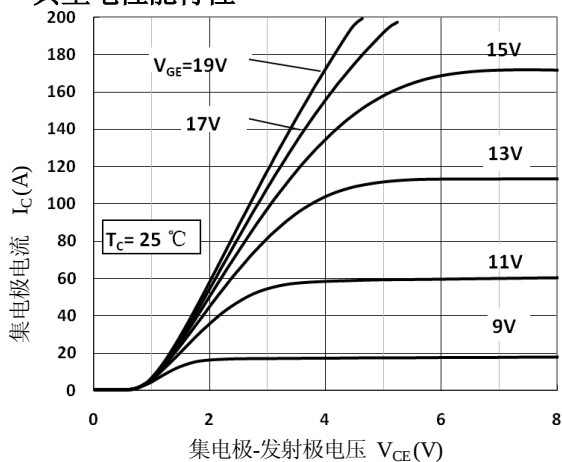
图 1. 输出特性
