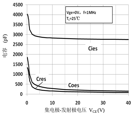
图 7. 电容特性
