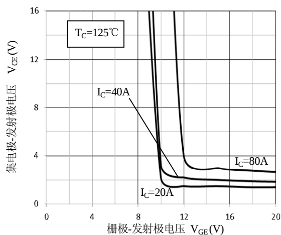
图 6. 饱和压降— V_{GE} 特性
