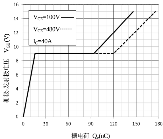
图 14. 栅电荷特性
