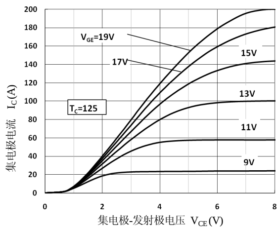
图 2. 输出特性
