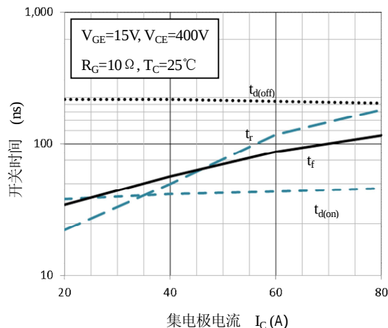
图 10. 开关时间— I_C 特性
