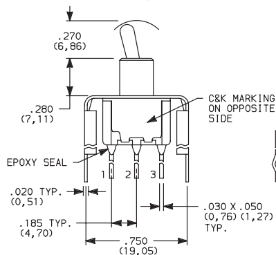
7101MD9_BE SPDT
