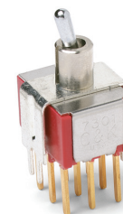
7301MD9_BE 3PDT
