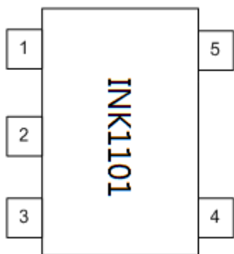
SOT-23-5
