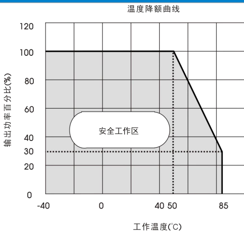
图 2 K78U24-300R3(L) (Vin≥60V)
