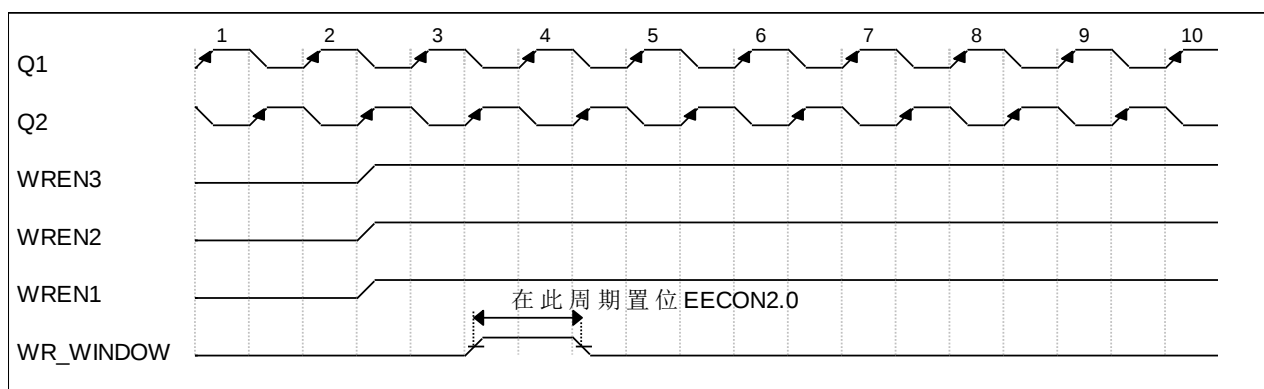
图 8.1 软件编程数据 EEPROM 时序
