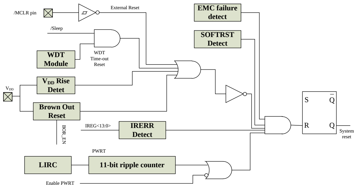
图 4.1 复位框图
