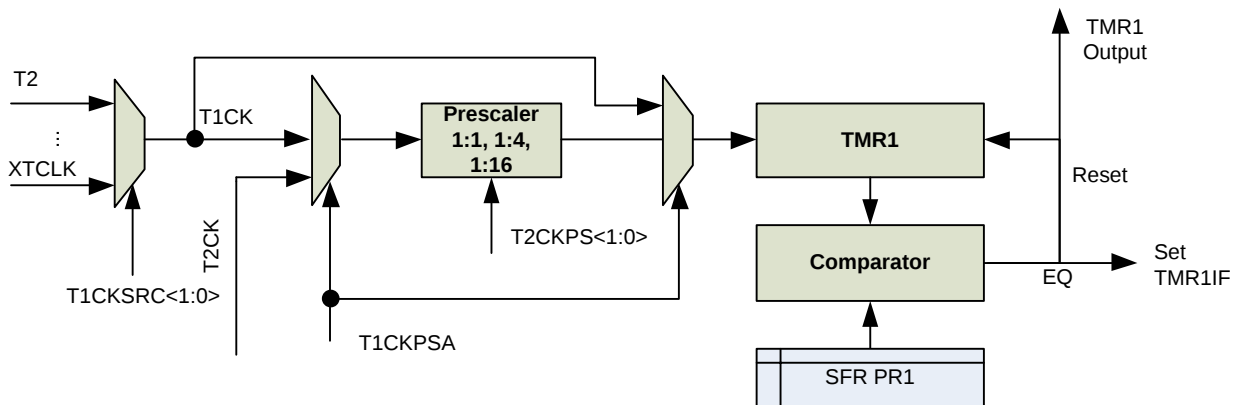
图 11.1 定时器 1 框图
