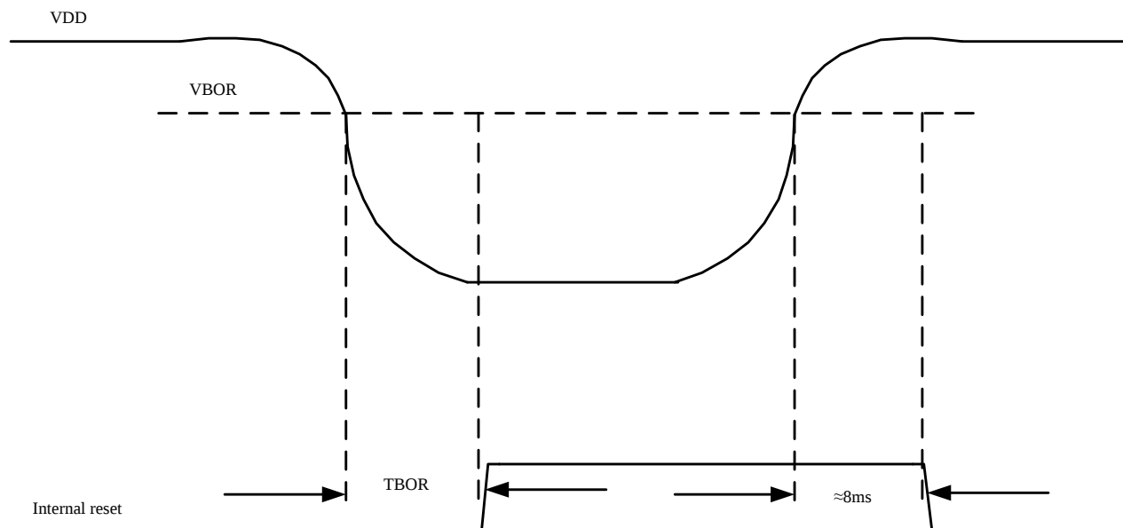
图 4.6 BOR 复位
