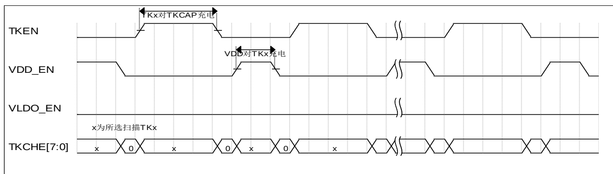
图 16.4 充电模式下 TOUCH 功能时序图
