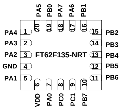
图 1.7 QFN20 脚位
