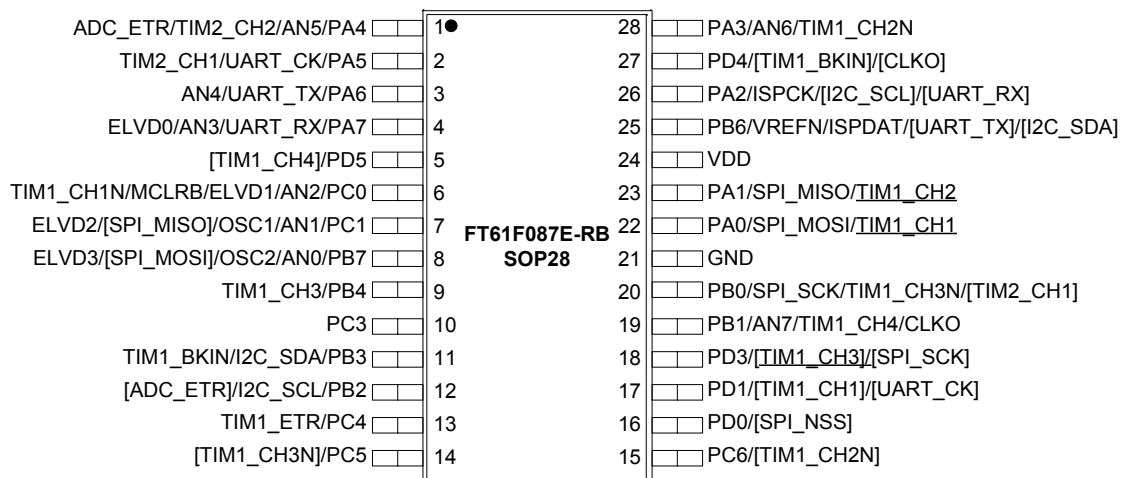
图 1.4 SOP28 脚位 2
