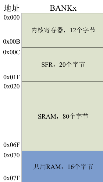
图 3.1 存储区构成
