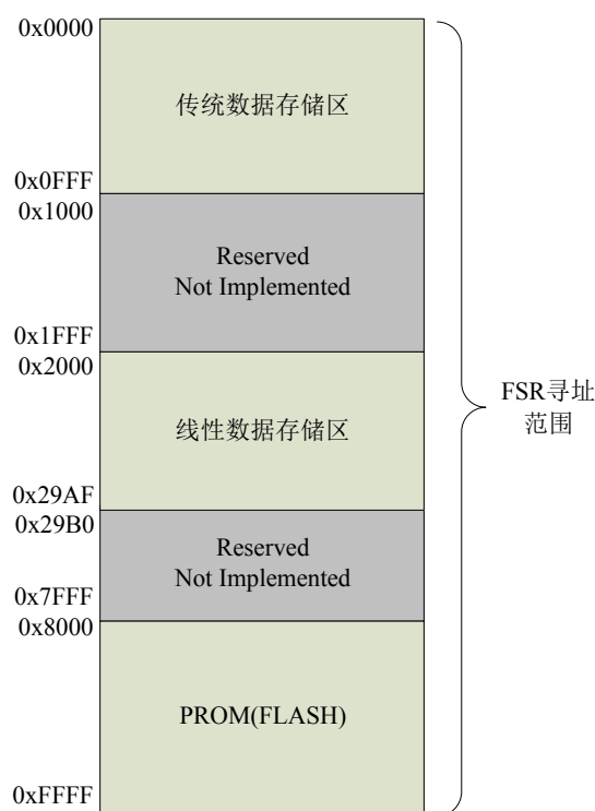
图 3.4 间接寻址
