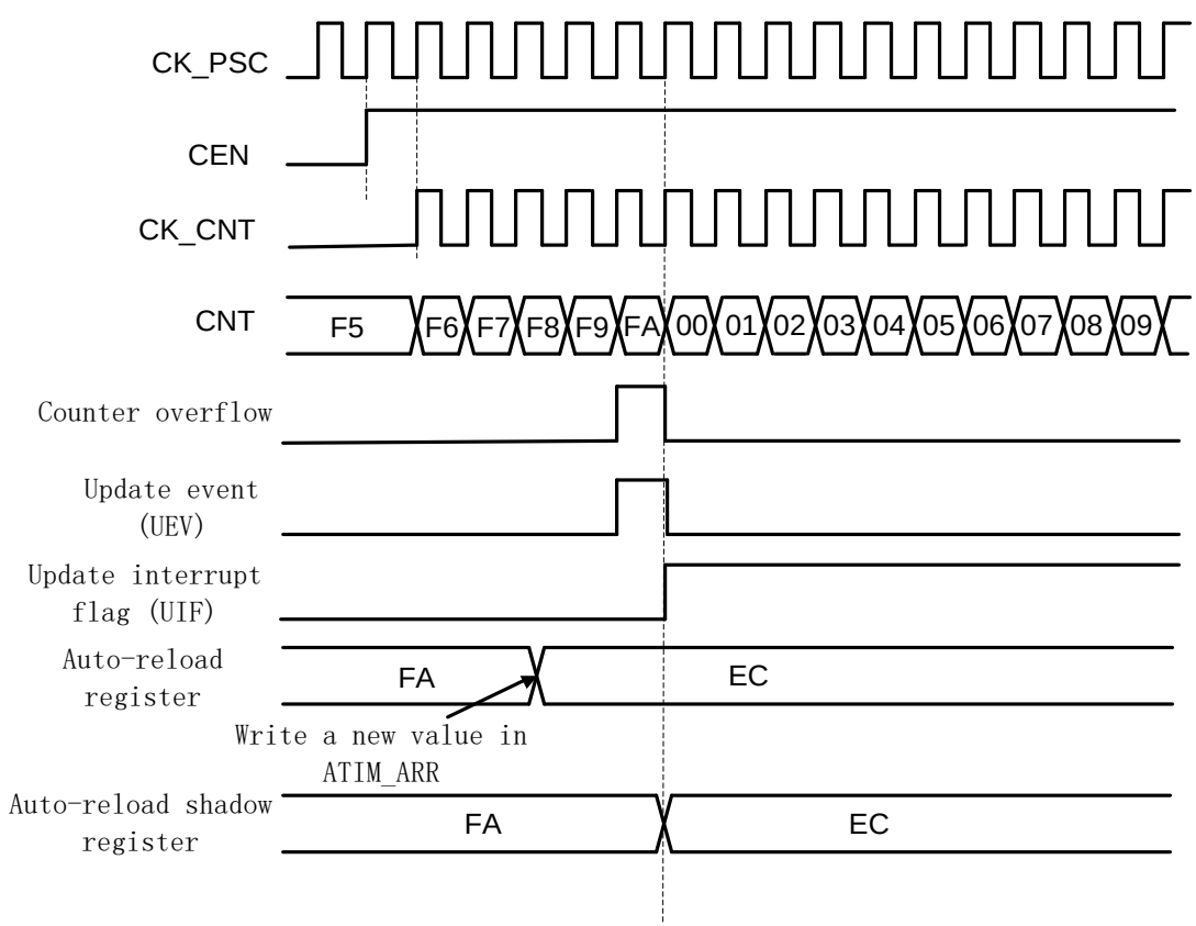
图 28-7ARPE=1（ARR 预装载）时的更新事件
