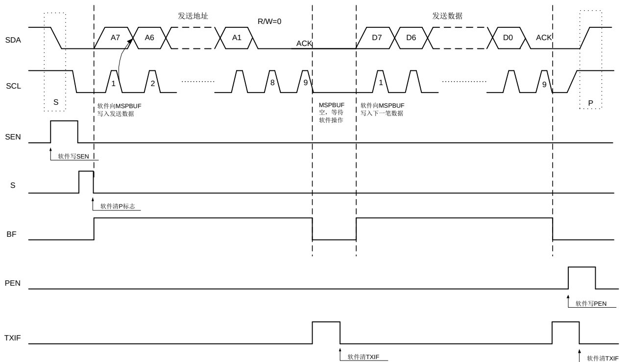
图 19-9I2C 主机对 7 位地址从机发送数据流程图
