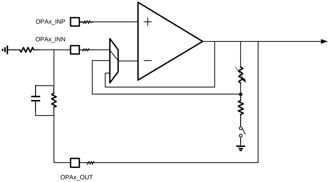
图 16-4OPA 独立模式
