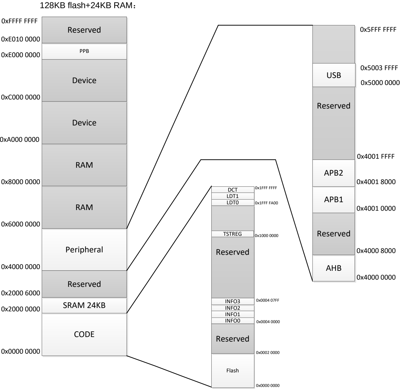
图 7-3FM33LC02x 总线地址
