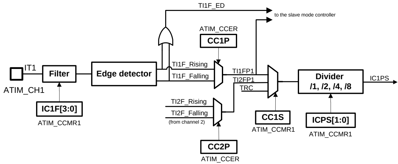
图27-23捕捉/比较通道(通道1输入部分)
