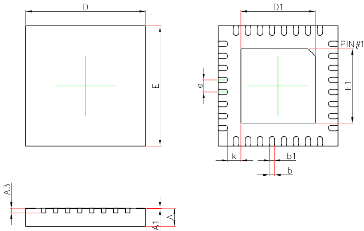
图 2-11QFN32 封装尺寸图
