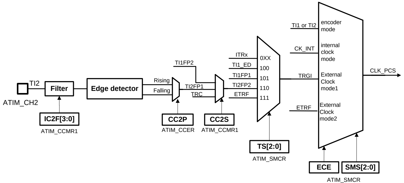
图 26-18 TI2 外部时钟连接例子
