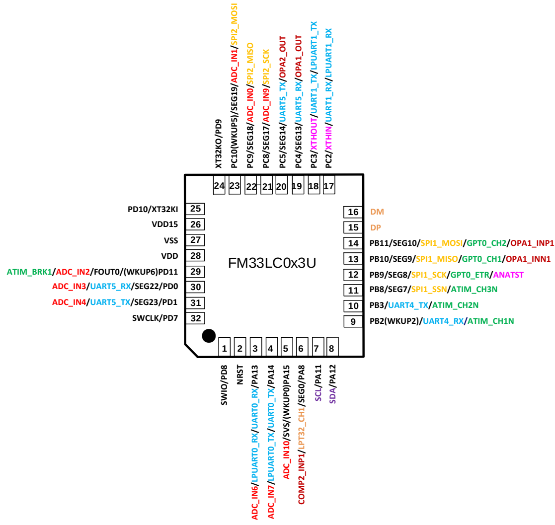
图 2-6FM33LC0x3U QFN32 封装图
