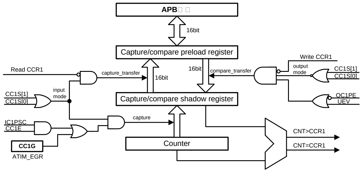
图27-24捕捉/比较通道1的主电路
