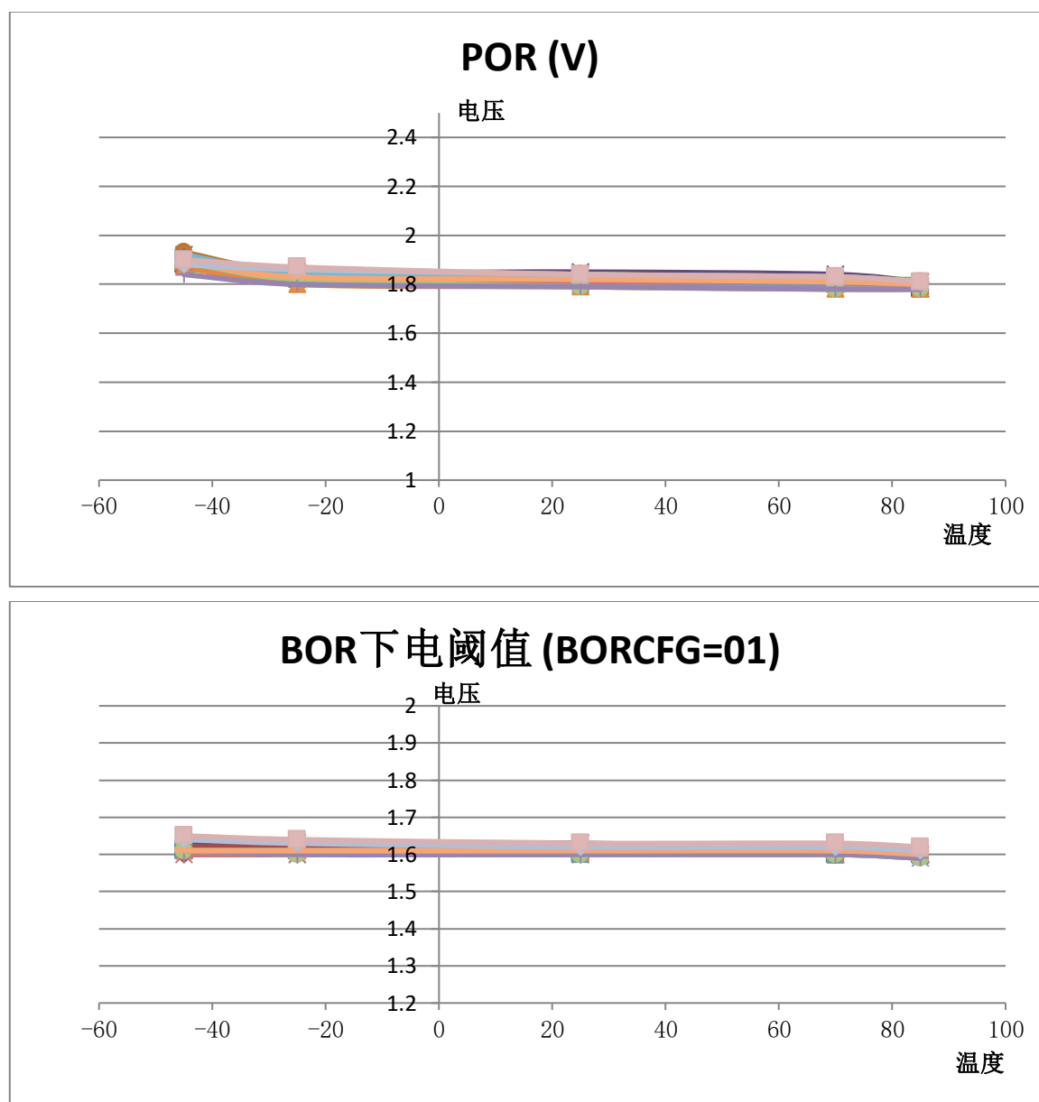
上电复位释放阈值-温度曲线（基于特征参数提取，仅供设计参考）
