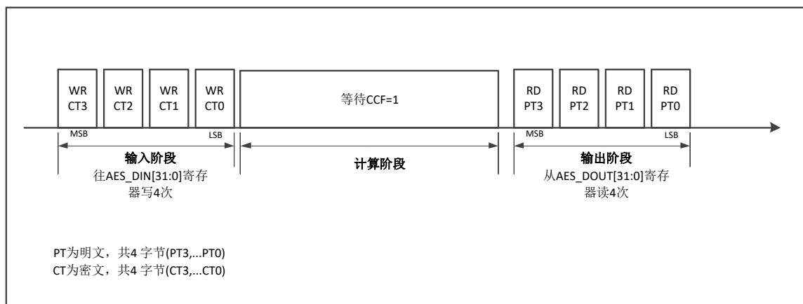
图 14-16 模式 4 示意图
