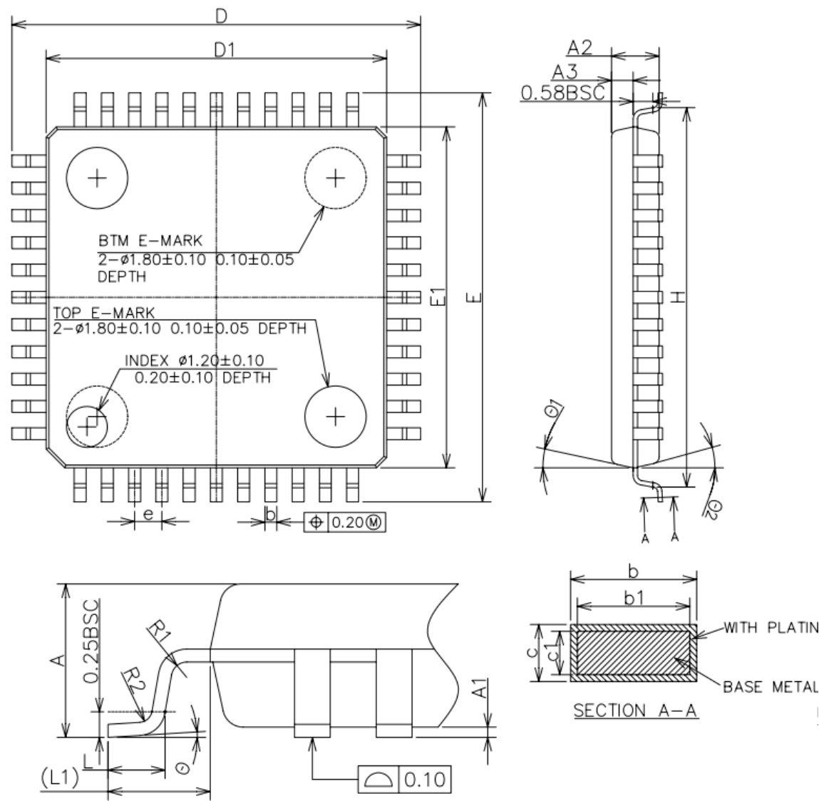
图 2-10LQFP44 封装尺寸图
