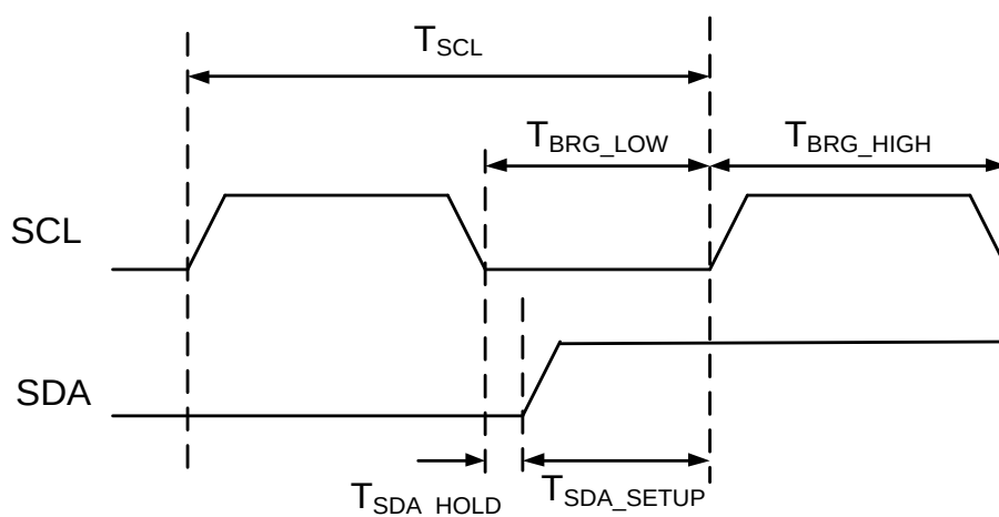
图 19-21 主机时序控制
