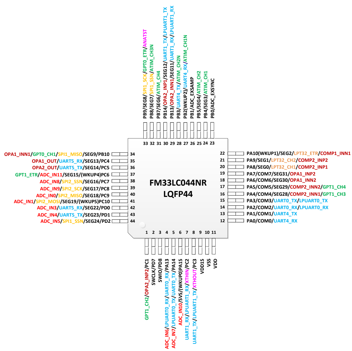
图 2-4FM33LC0x4NR LQFP44 封装图
