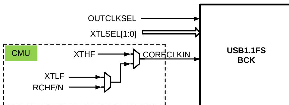
图 11-2USB PHY 参考时钟源选择
