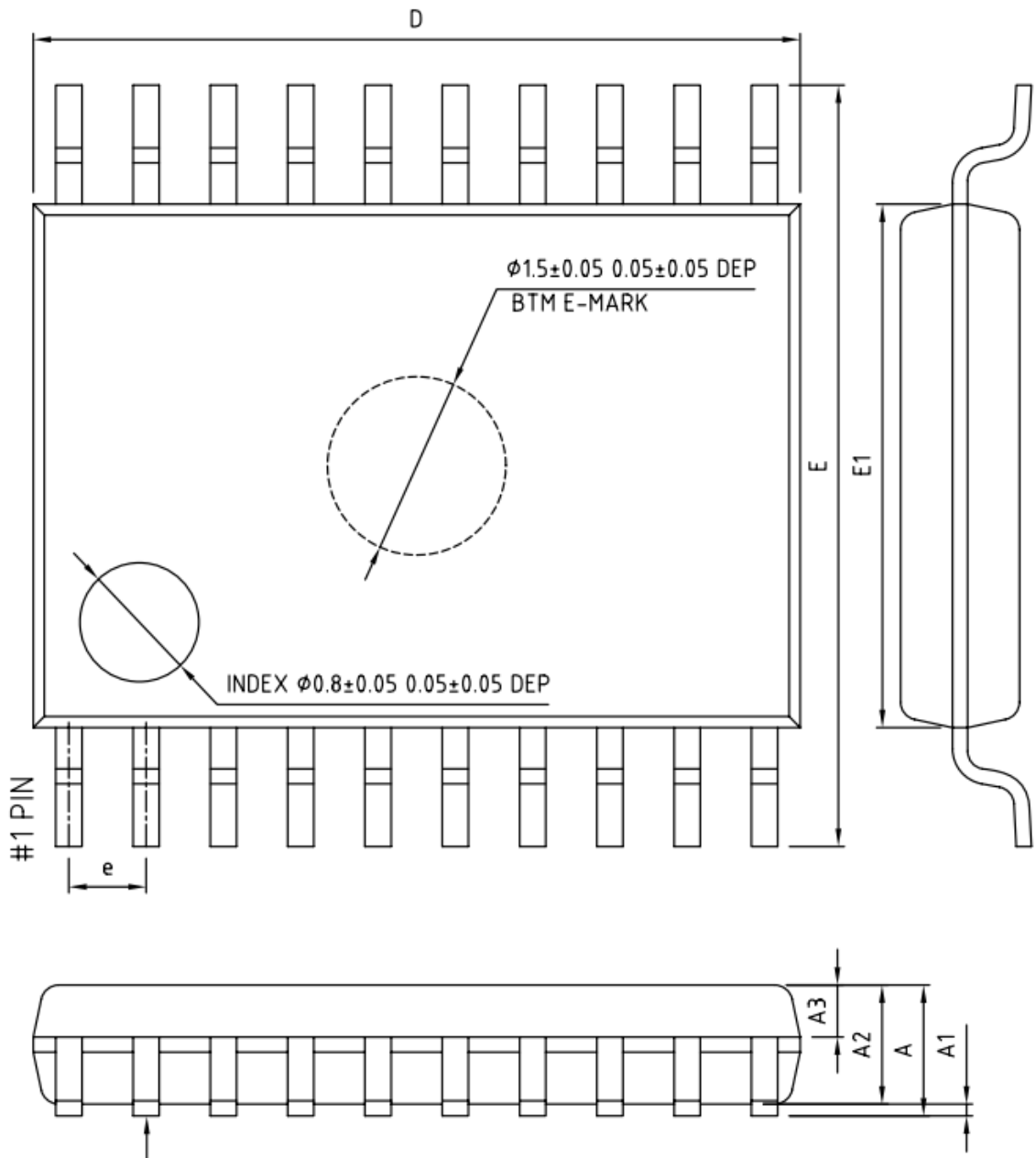
图 2-12TSSOP20 封装尺寸图
