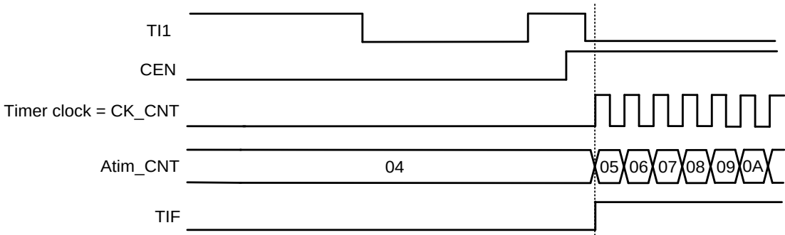
图27-35触发器模式下的时序
