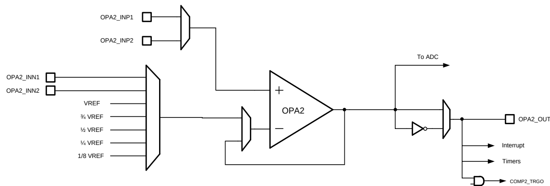
图 16-2OPA2 电路框图
