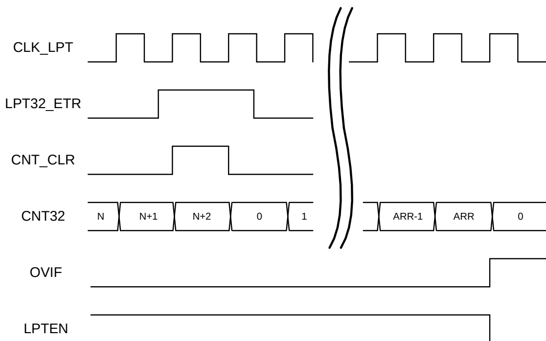
图 29-4TimeOut 模式
