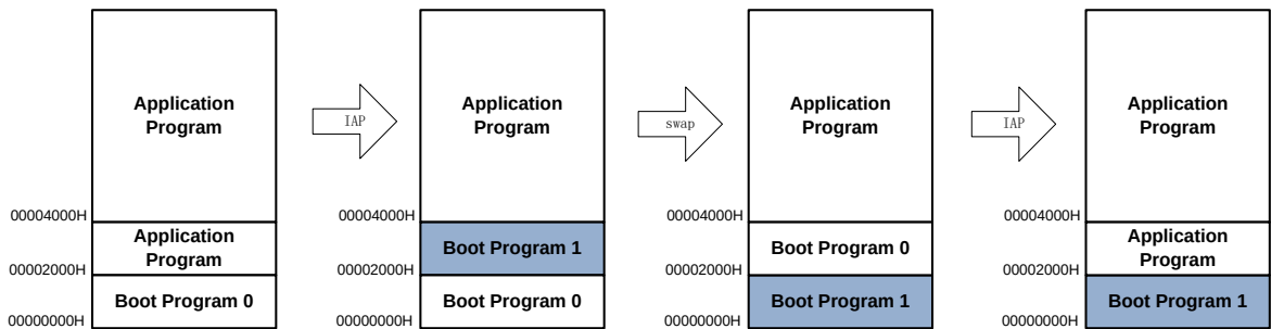
图 7-4Bootswap 示意图
