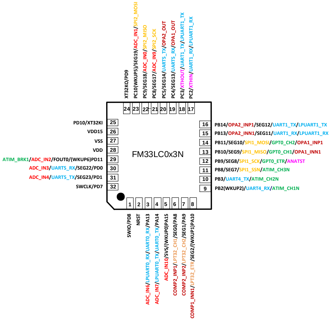
图 2-5FM33LC0x3NQFN32 封装图
