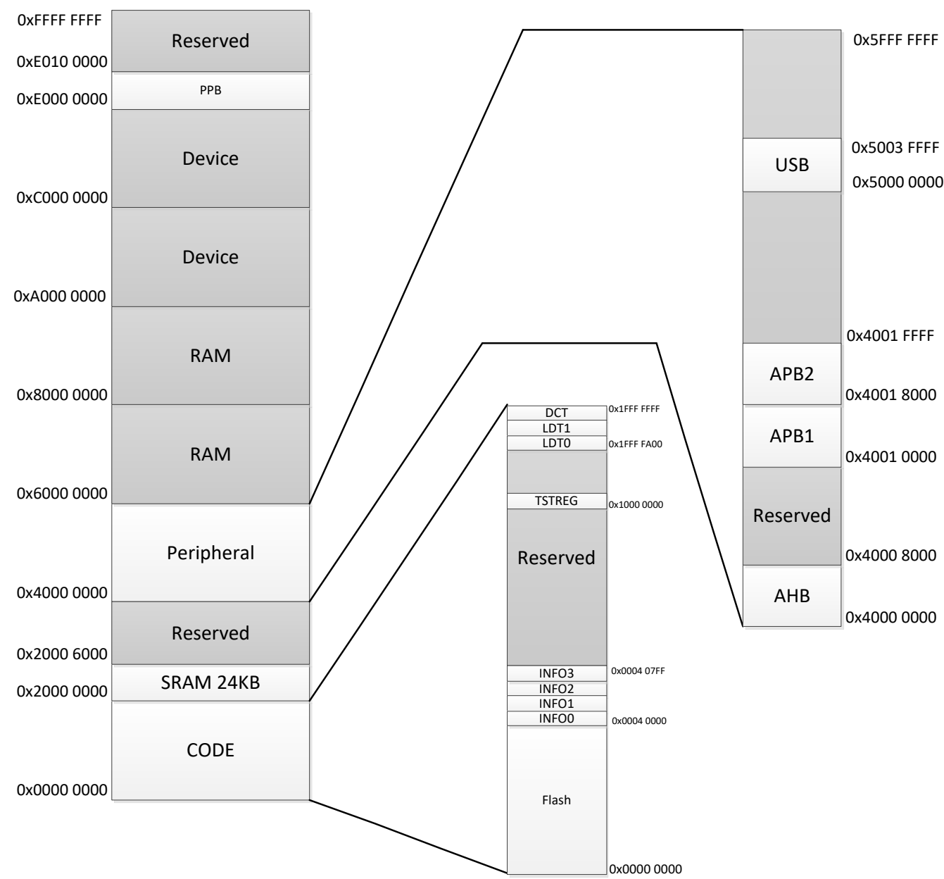
图 7-2FM33LC04x 总线地址
