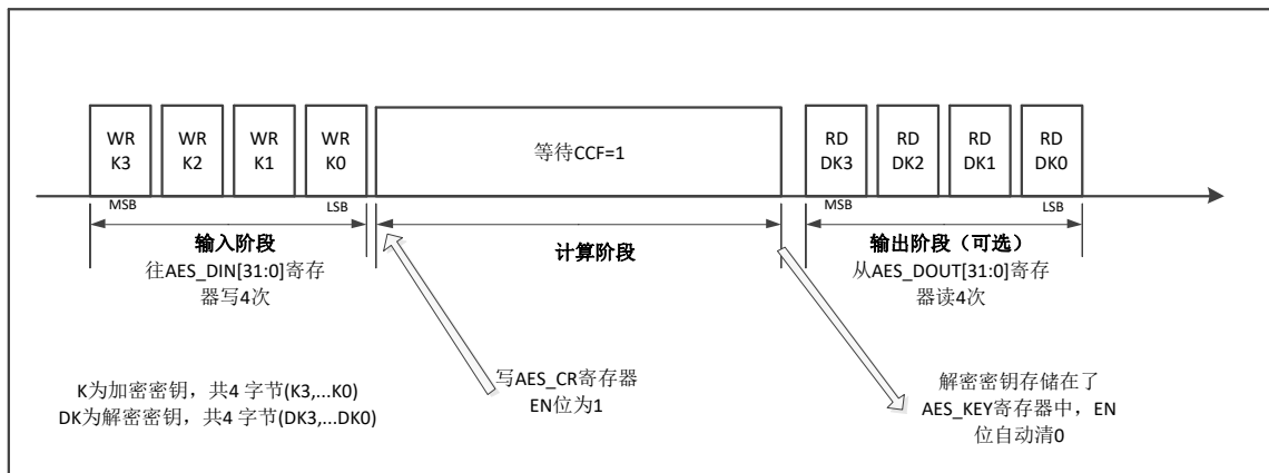
图 14-14 模式 2 示意图
