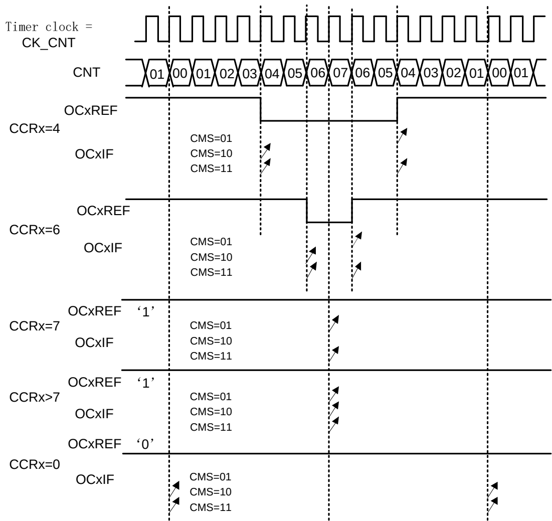
图27-29中央对齐的PWM波形(APR=7)
