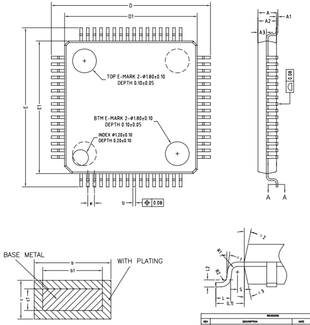
图 2-8 LQFP64 封装尺寸图
