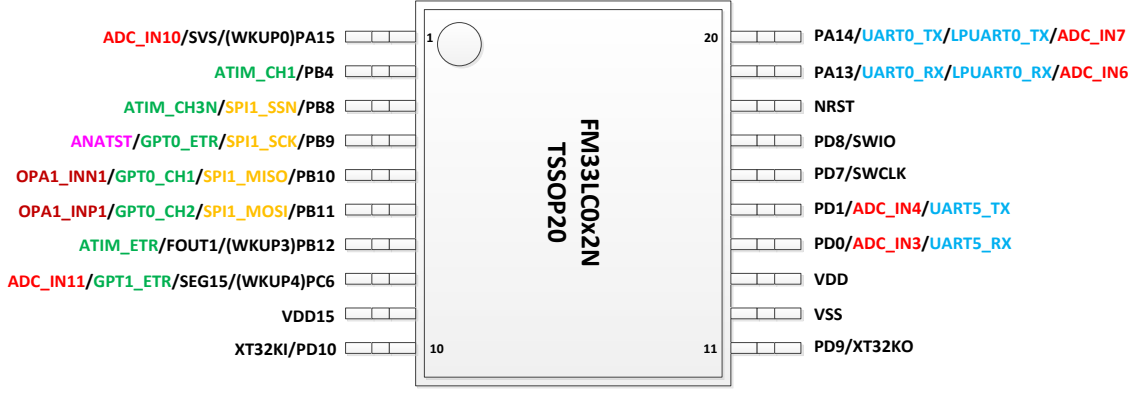
图 2-7FM33LC0x3NTSSOP20 封装图
