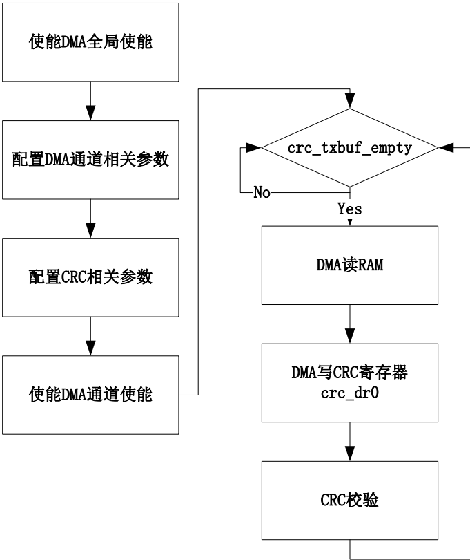
图25-2使用DMA对RAM中的数据进行CRC运算
