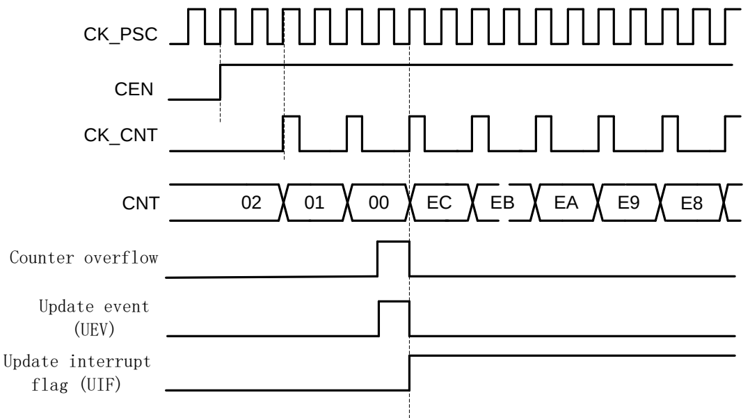
图 26-9 向下计数，内部时钟 2 分频
