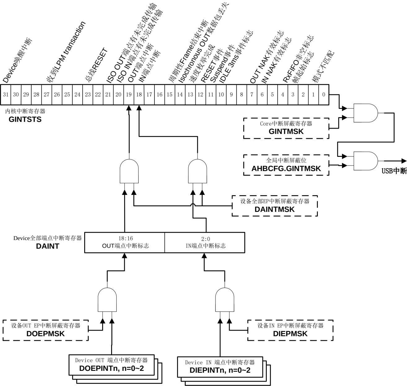
图 33-3USB 外设中断示意图
