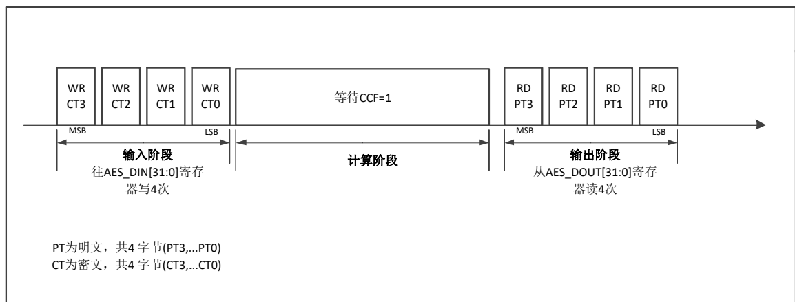
图 14-15 模式 3 示意图
