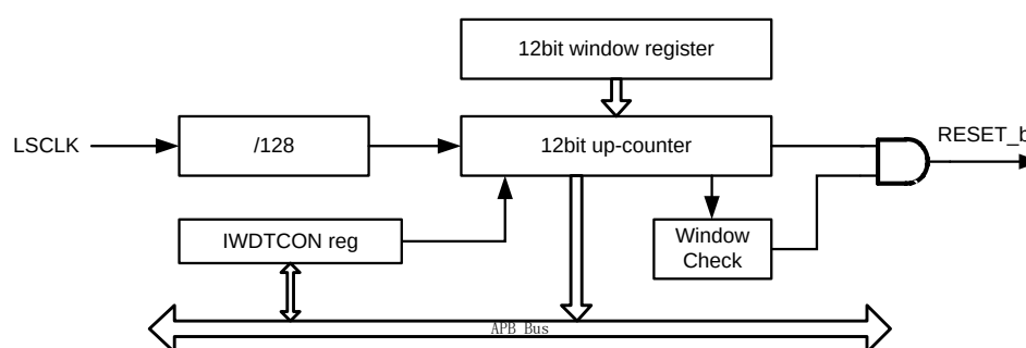
图 9-1 IWDG 结构框图
