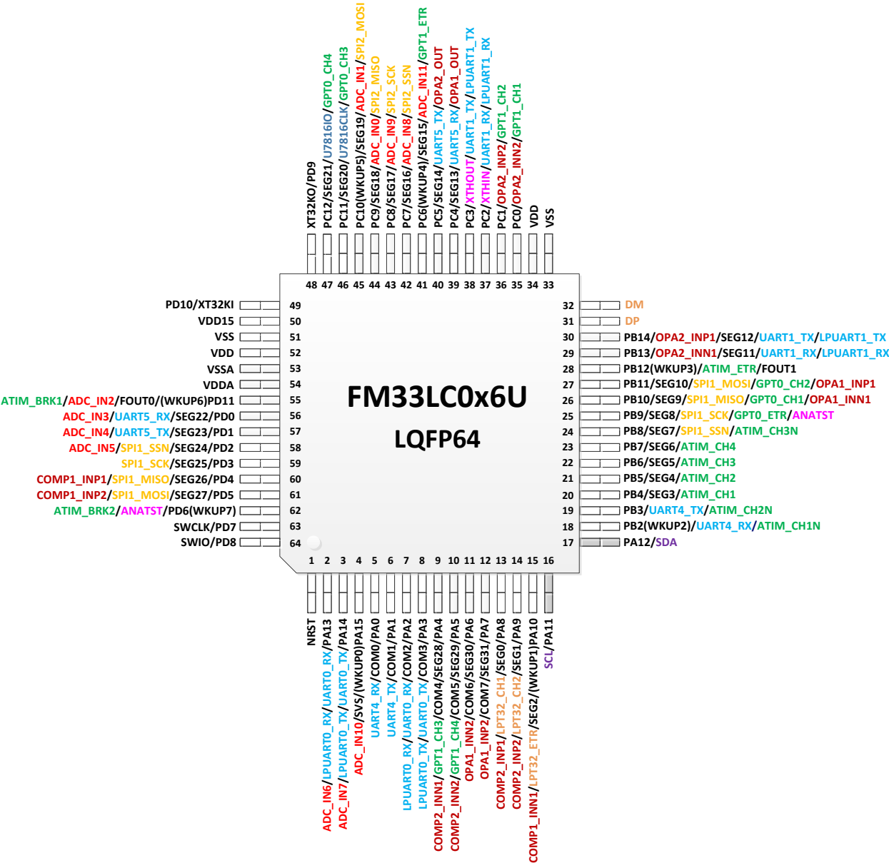
图 2-1FM33LC0x6U LQFP64 封装图
