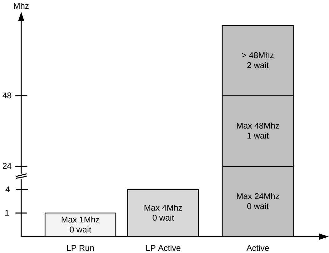
图 4-2 功耗模式与系统主频
