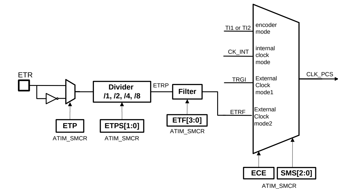
图 27-20 外部触发输入框图
