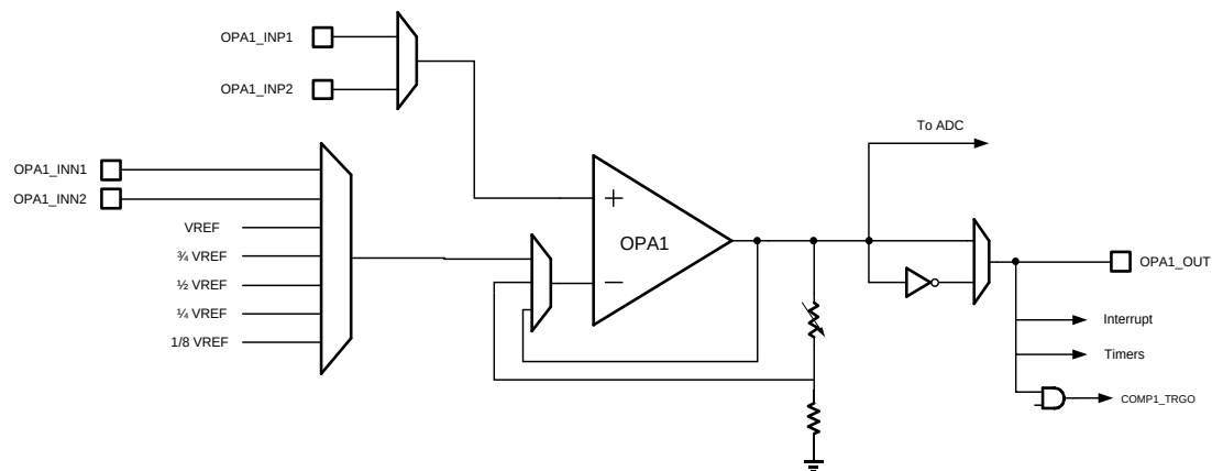
图 16-1OPA1 电路框图
