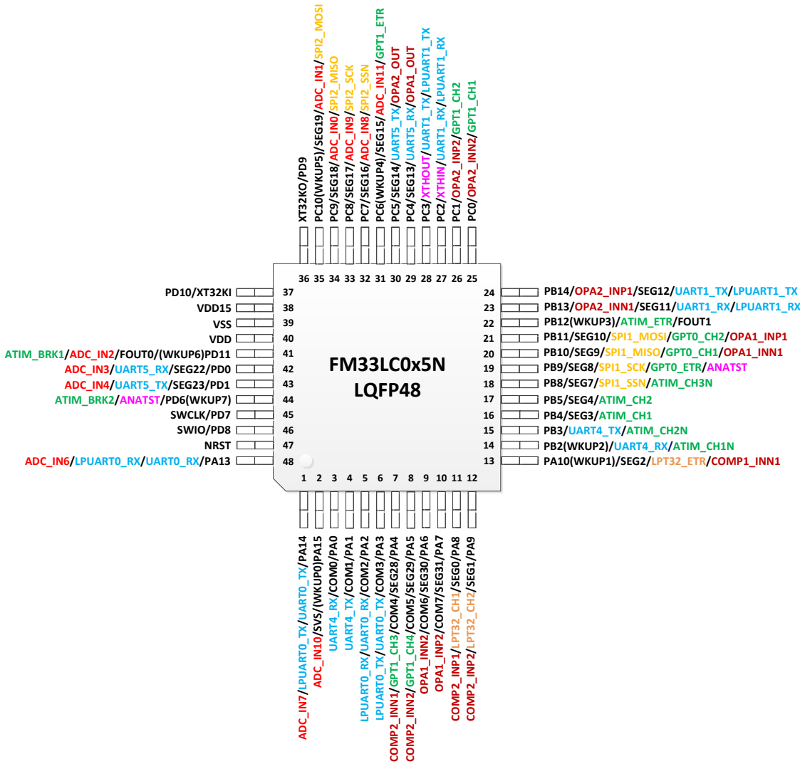
图 2-3FM33LC0x5N LQFP48 封装图
