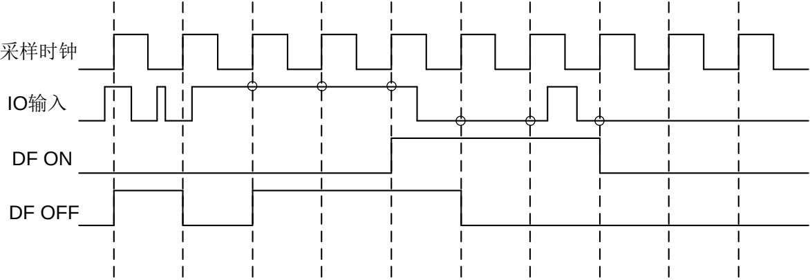
图 34-5 引脚输入数字滤波
