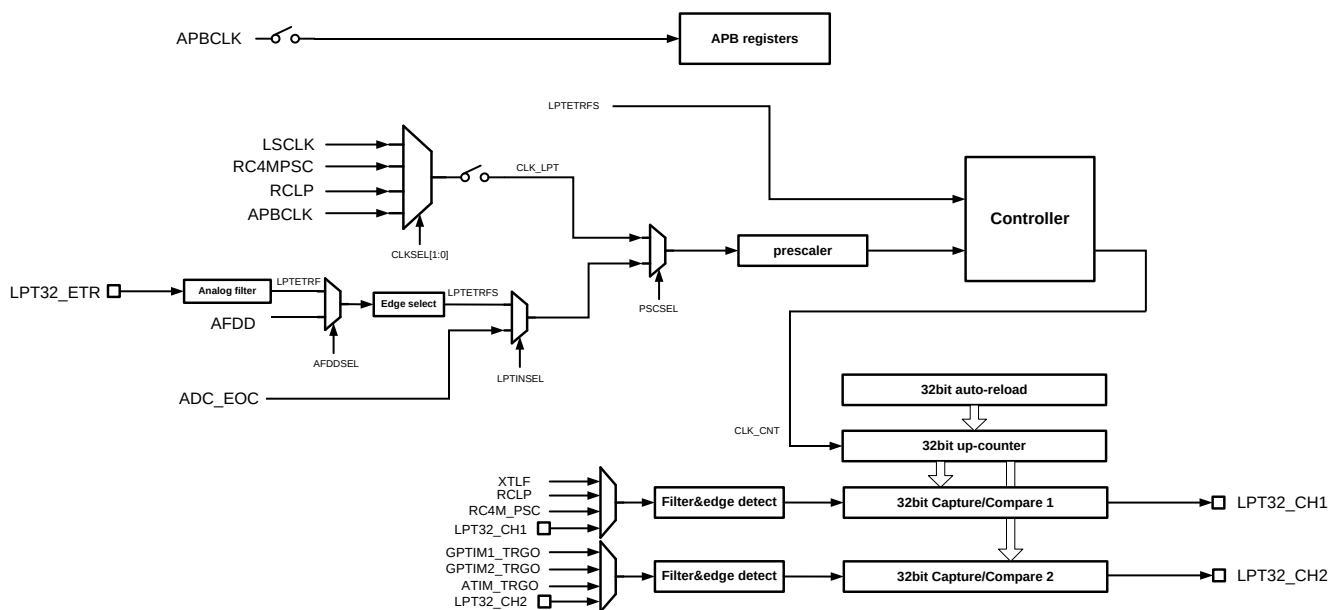
图 29-1LPTIM32 结构框图
