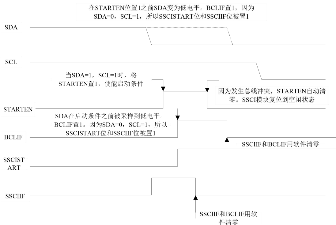
图9.21 启动条件期间的总线冲突（仅 SDA）
