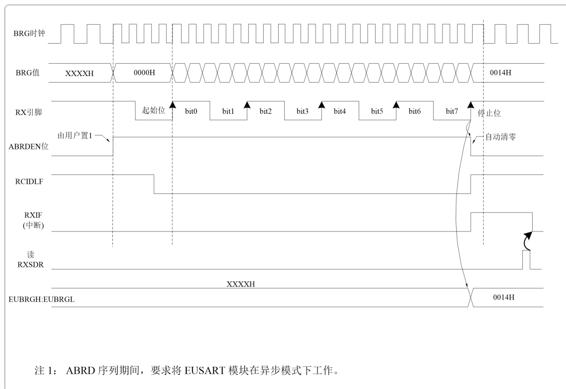
图 11.3 自动波特率检测
