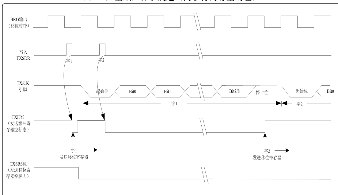
图 11.9 全双工异步发送（两字符间有空闲位）
