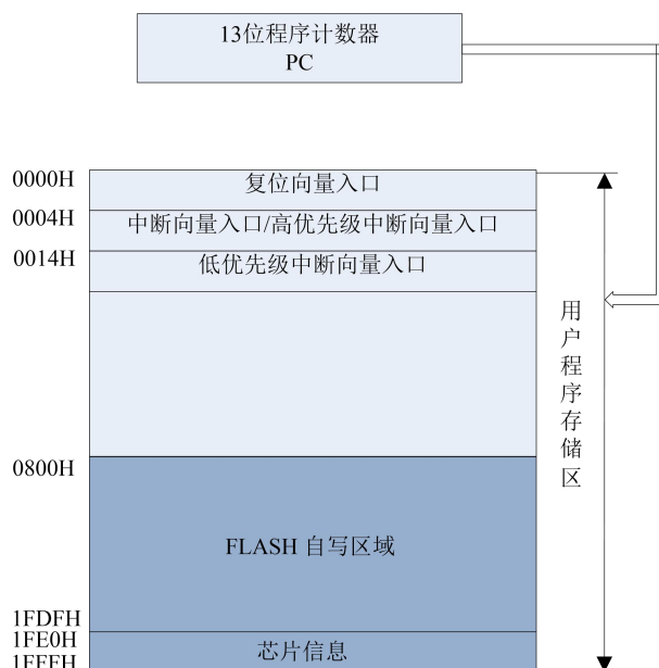
图 3.3 KF8A100ENG 程序存储器映射
