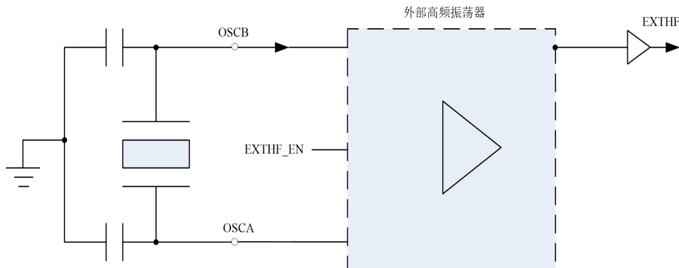
图 1.3 EXTHF 原理图
