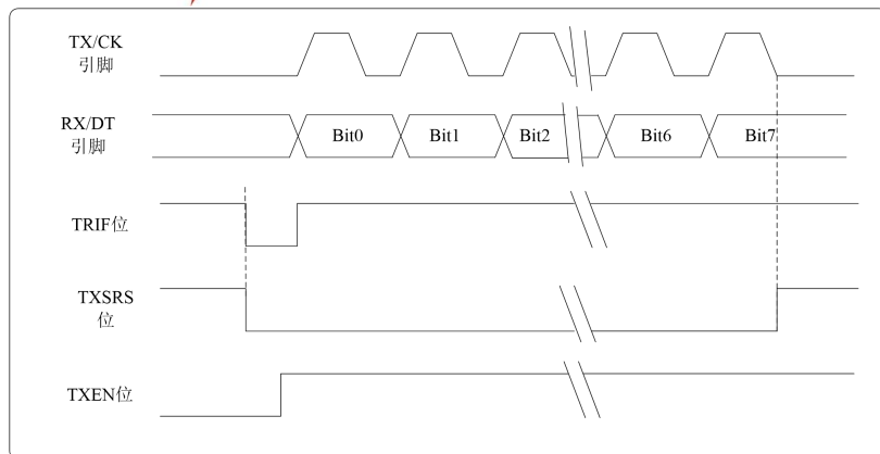
图 11.14 半双工同步发送（通过 TXEN）
