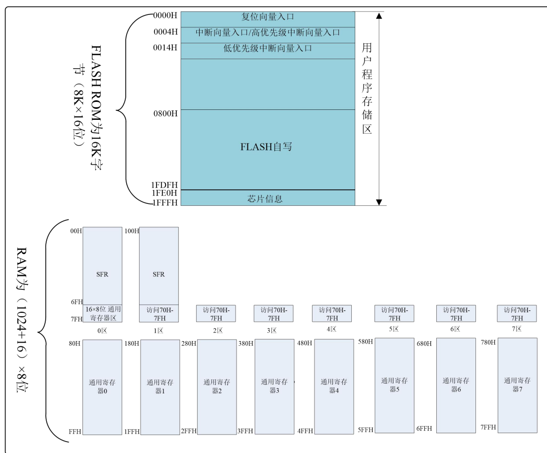
图 3.1 KF8A100ENG 存储器组织图
