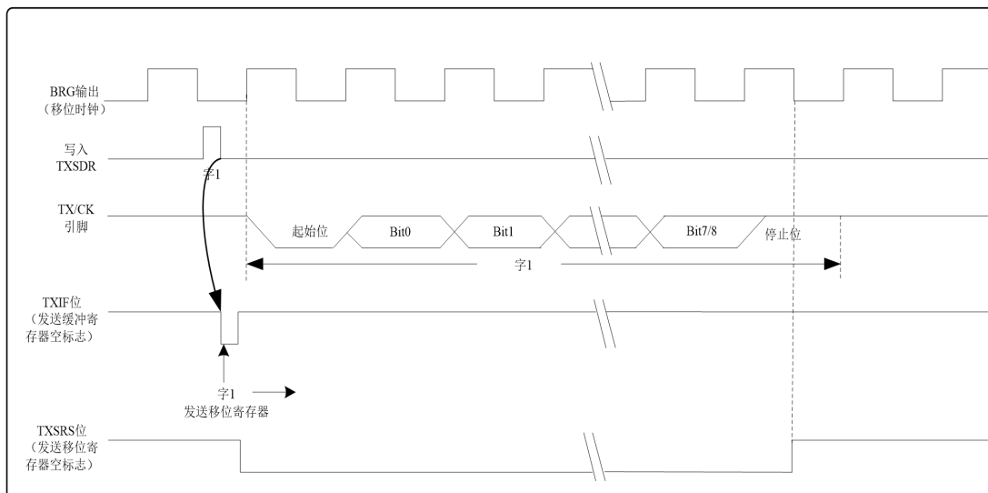
图 11.9 全双工异步发送（两字符间有空闲位）
