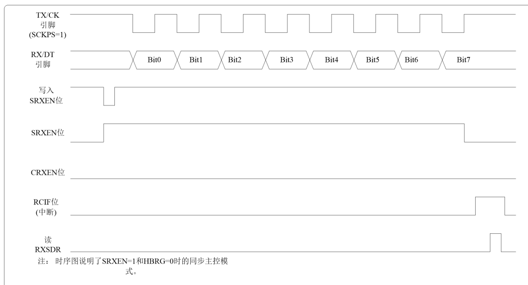
图 11.16 半双工同步接收（主控模式，SRXEN=1，SCKPS=1）
