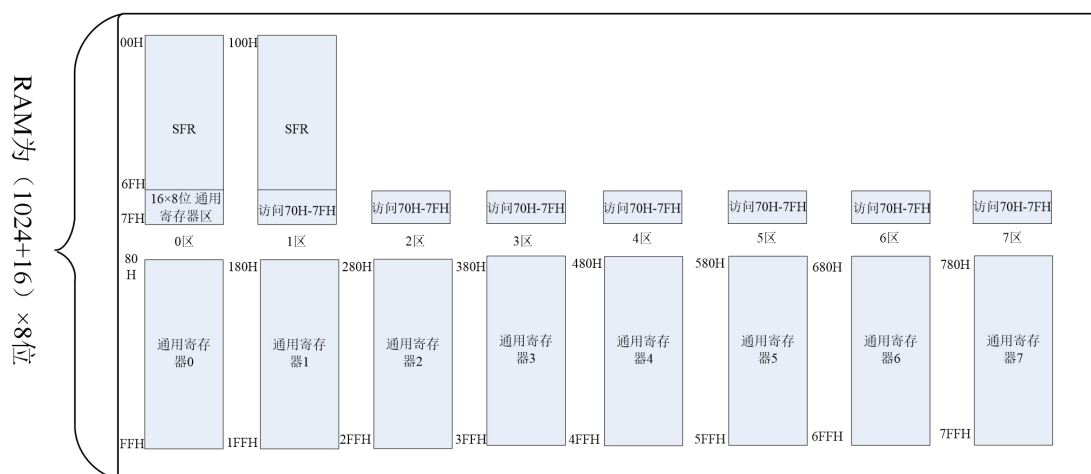
图 3.6 KF8A100ENG 数据存储器地址映射图
