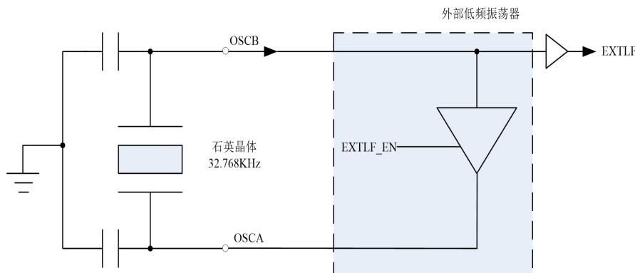
图 1.4 EXT LF 原理图
