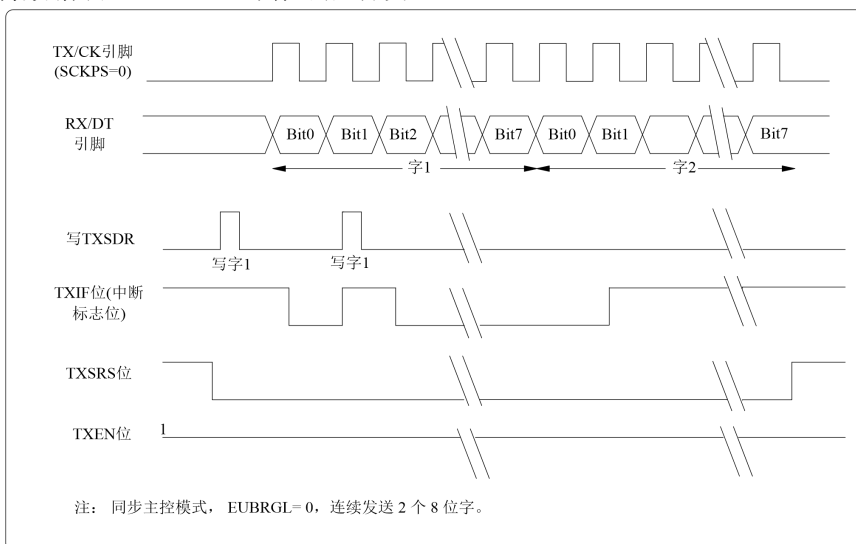
图 11.12 半双工同步发送 (SCKPS=0)
