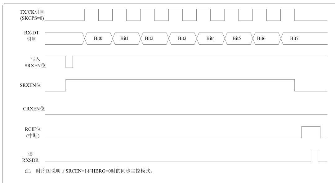
图 11.15 半双工同步接收（主控模式，SRXEN=1，SCKPS=0）
