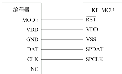
图 1.11 在线串行编程连接图
