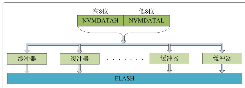
图 3.10 写操作
