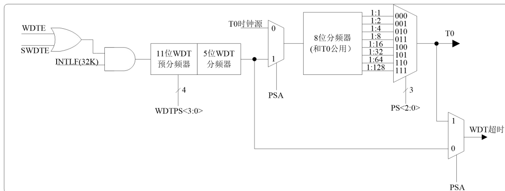
图 15.1 看门狗定时器框图
