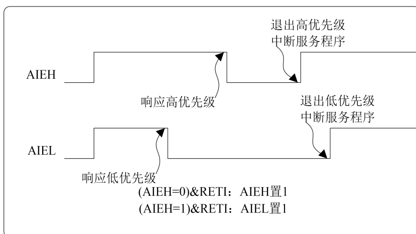
图 5.1 中断优先级工作原理图
