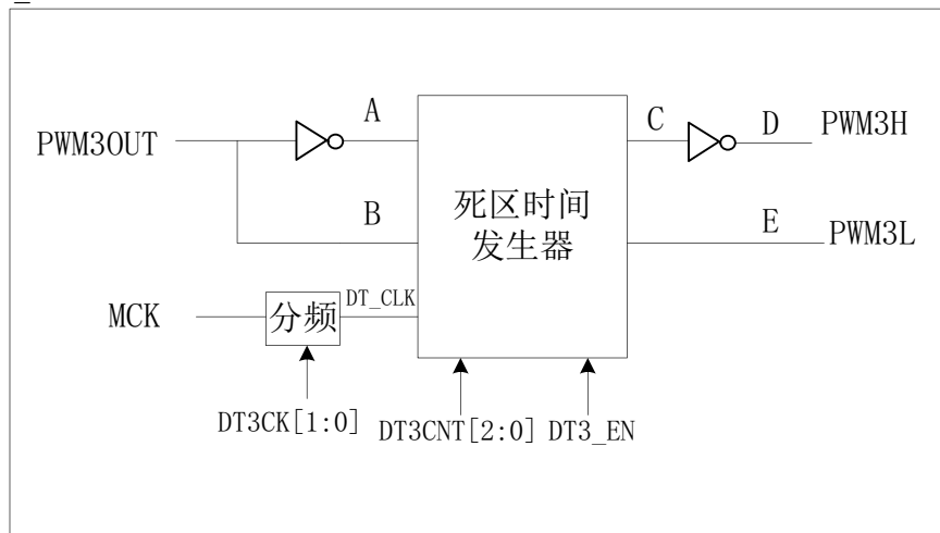
图13 互补式 PWM 输出方框图
