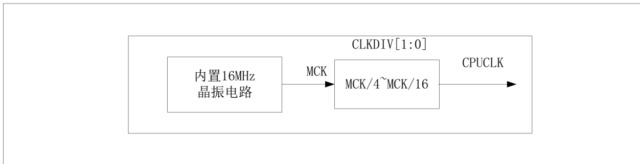
图4 GB2719 振荡器状态框图
