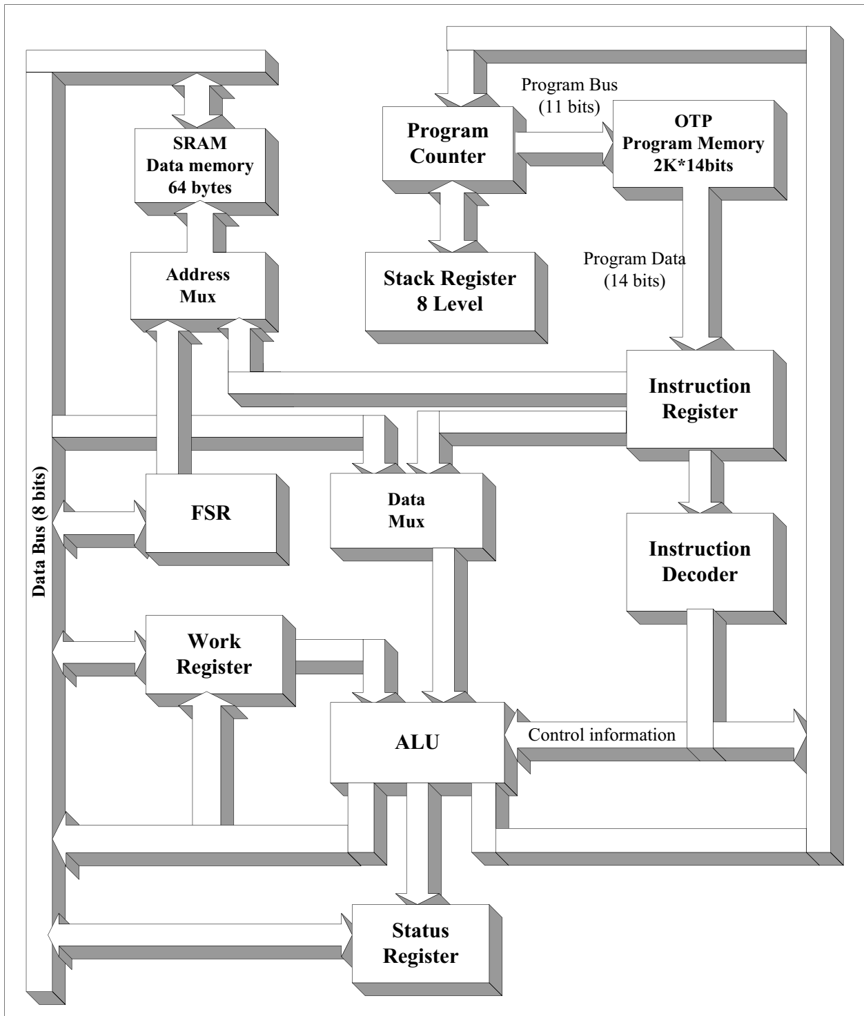
图1 GB2719 CPU 核的功能模块图
