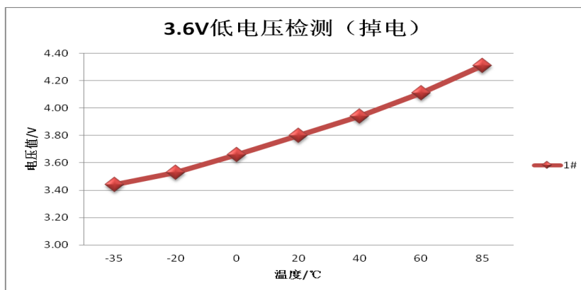
图20 3.6V 低电压复位温度特性
