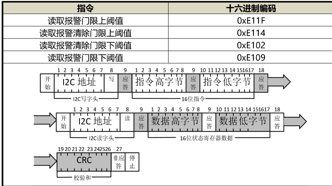
图 12.13-1 读取警报门限指令（白色块由微控制器控制，传感器响应为灰色块）
