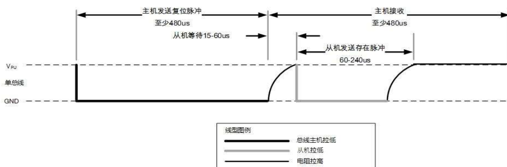
图 11.7-1 初始化时序
