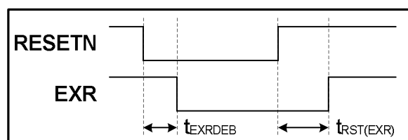
图 13. 外部复位 (EXR) 时序图
