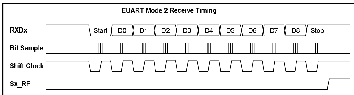
图 32. EUART 模式 2 接收时序图
