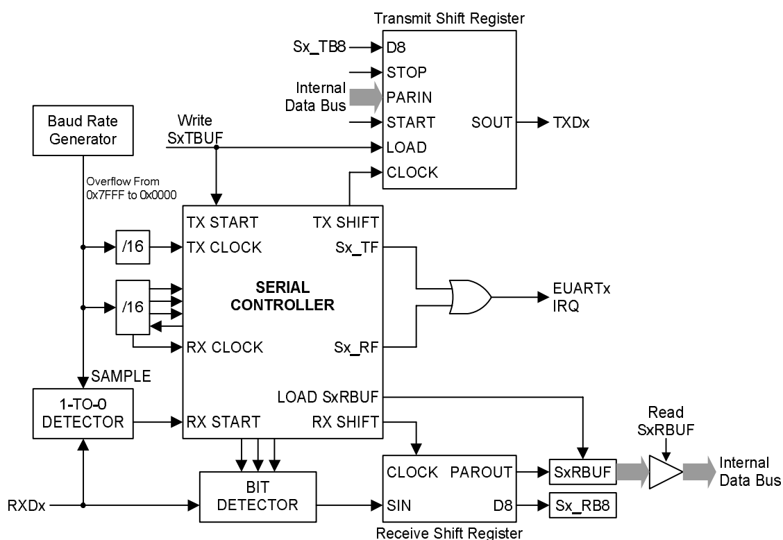
图 33. EUART 模式 2 结构框图
