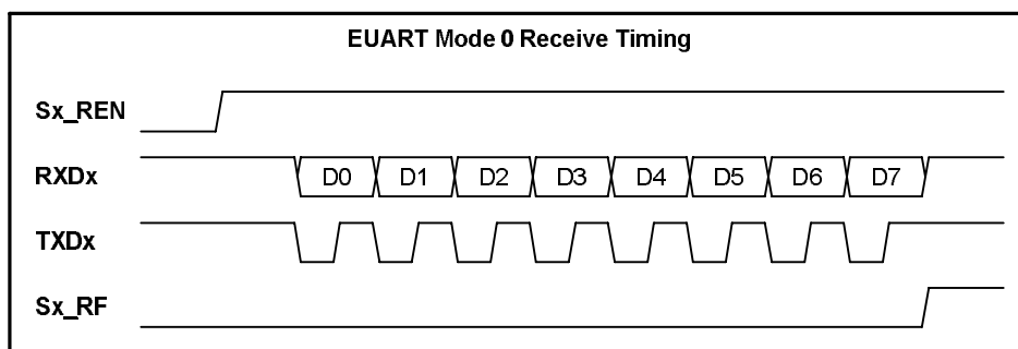
图 26. EUART 模式 0 接收时序图
