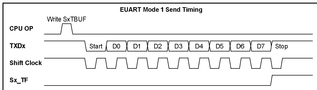
图 28. EUART 模式 1 发送时序图
