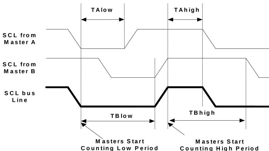
图 53. TWI 时钟同步
