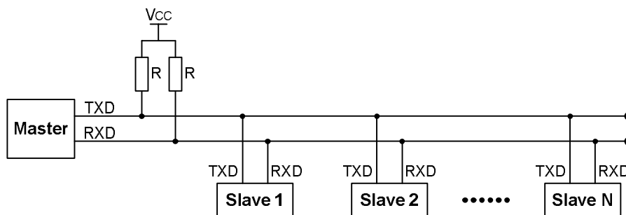
图 35. EUART 多机通讯连接图
