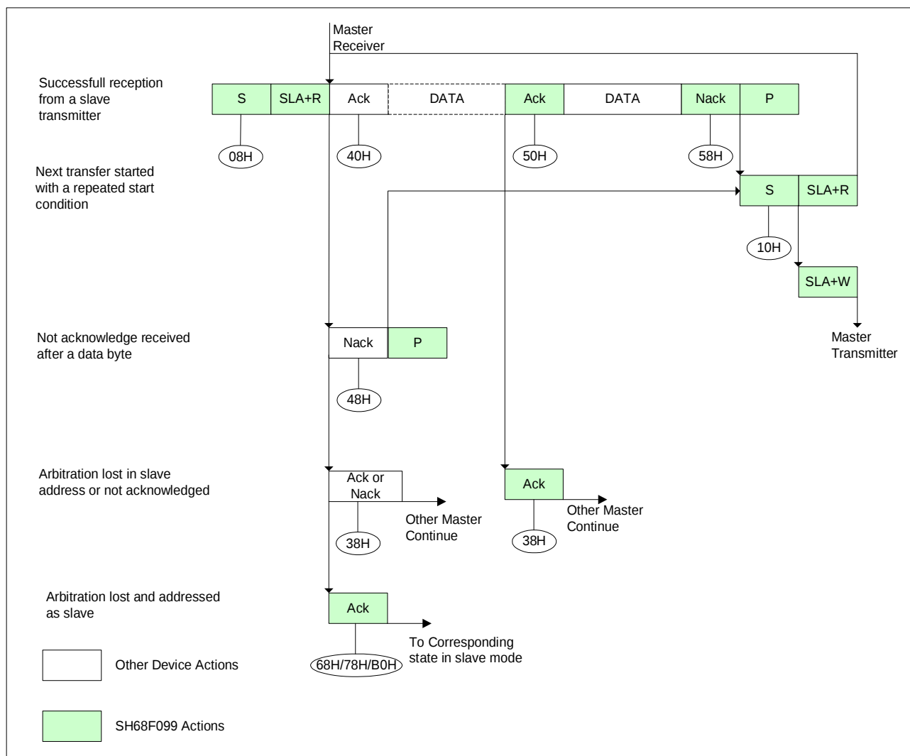
图 57. TWI 主机接收模式状态转换图
