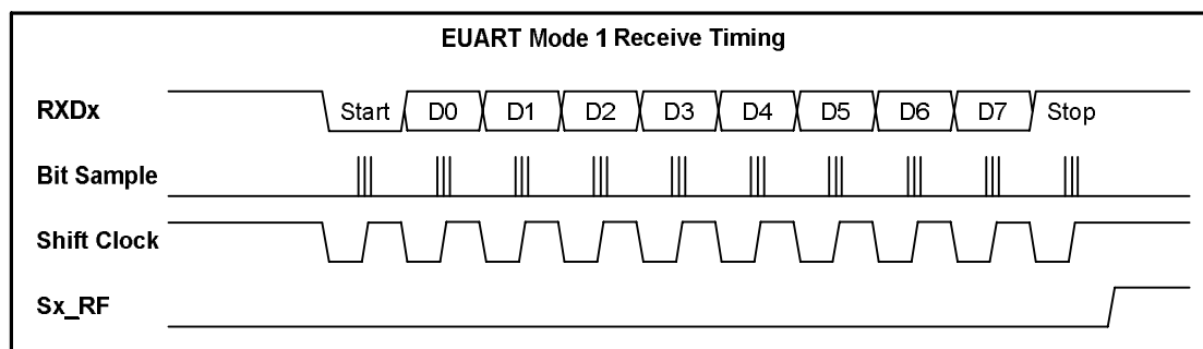
图 29. EUART 模式 1 接收时序图
