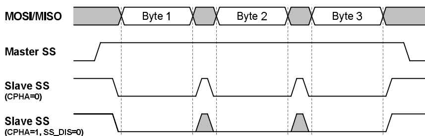
图 44. SS 引脚状态
