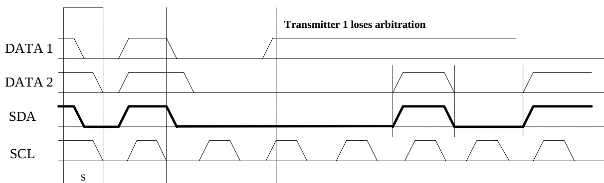
图 54. 总线仲裁
