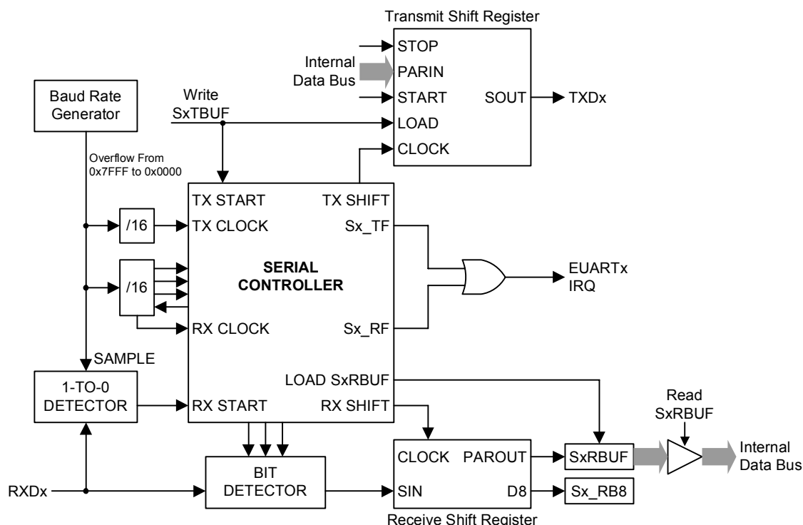
图 27. EUART 模式 1 结构框图
