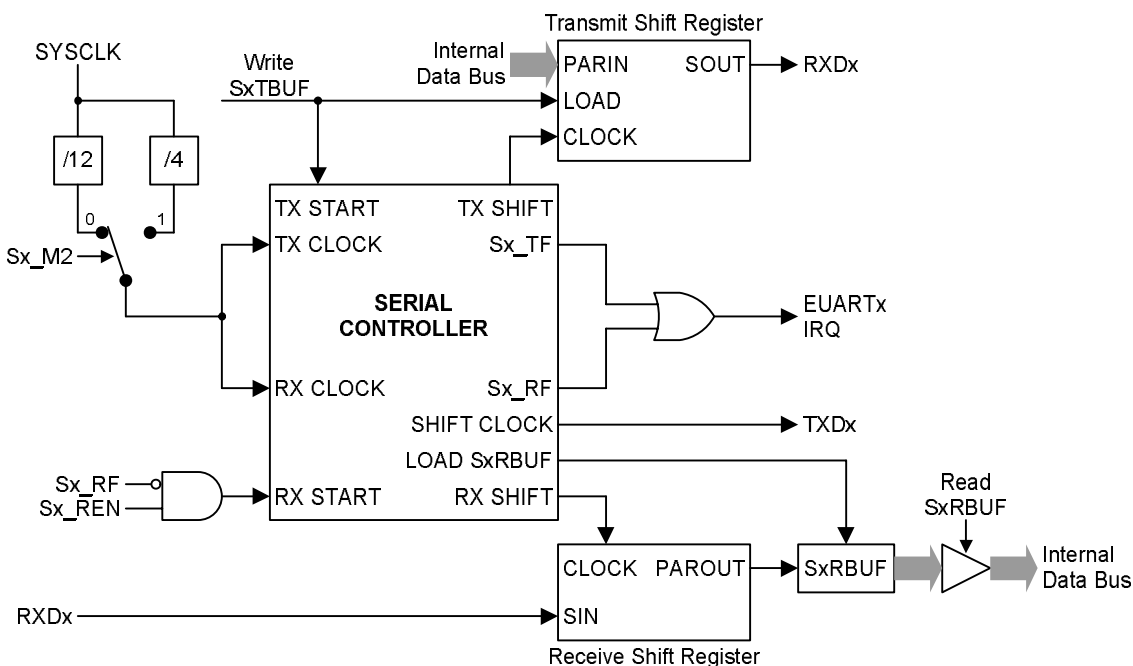
图 24. EUART 模式 0 结构框图
