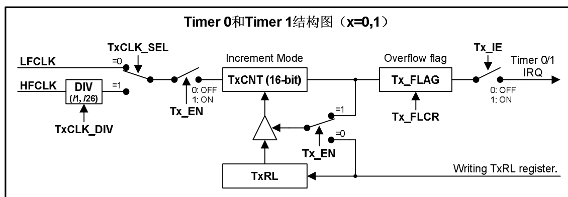
图 16. Timer 0/1 结构框图
