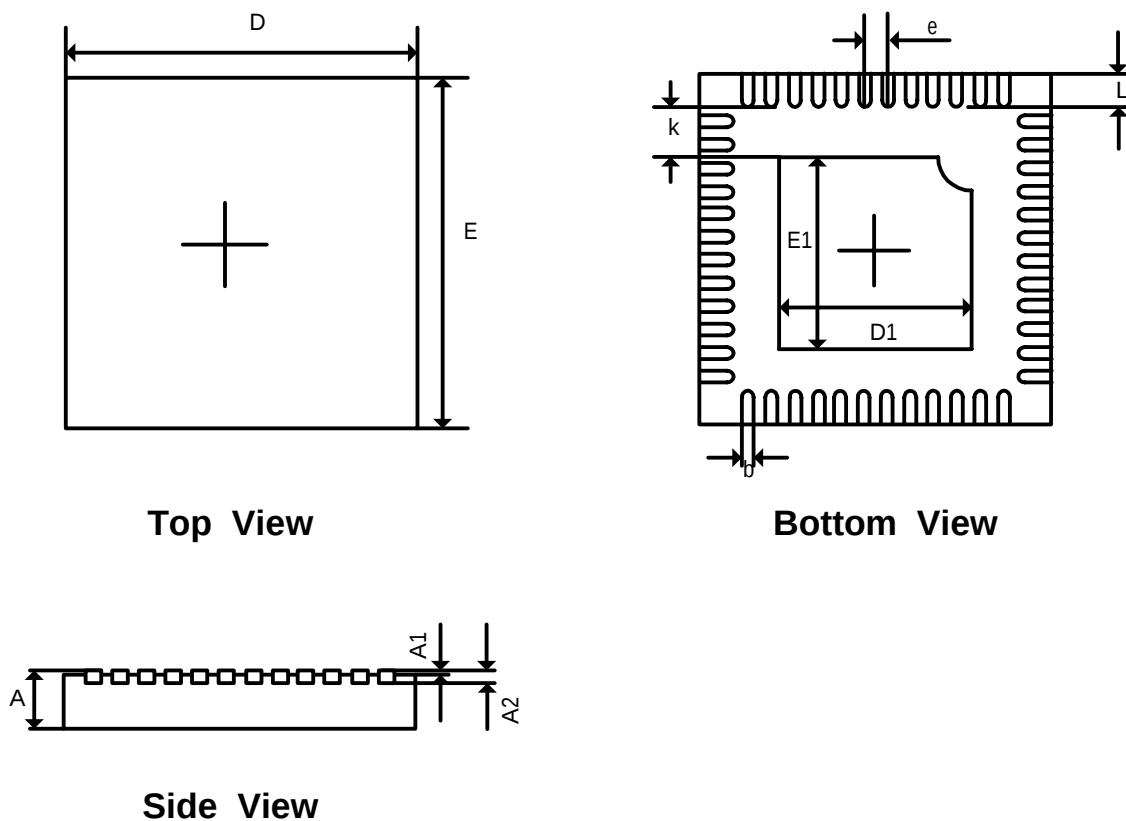
图 62. QFN48L(6x6) Outline Dimensions
