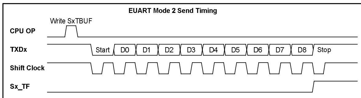
图 31. EUART 模式 2 发送时序图
