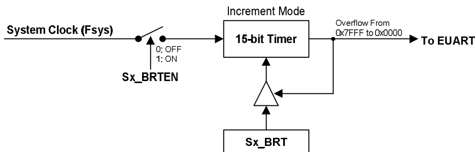
图 34. EUART 波特率发生器结构框图
