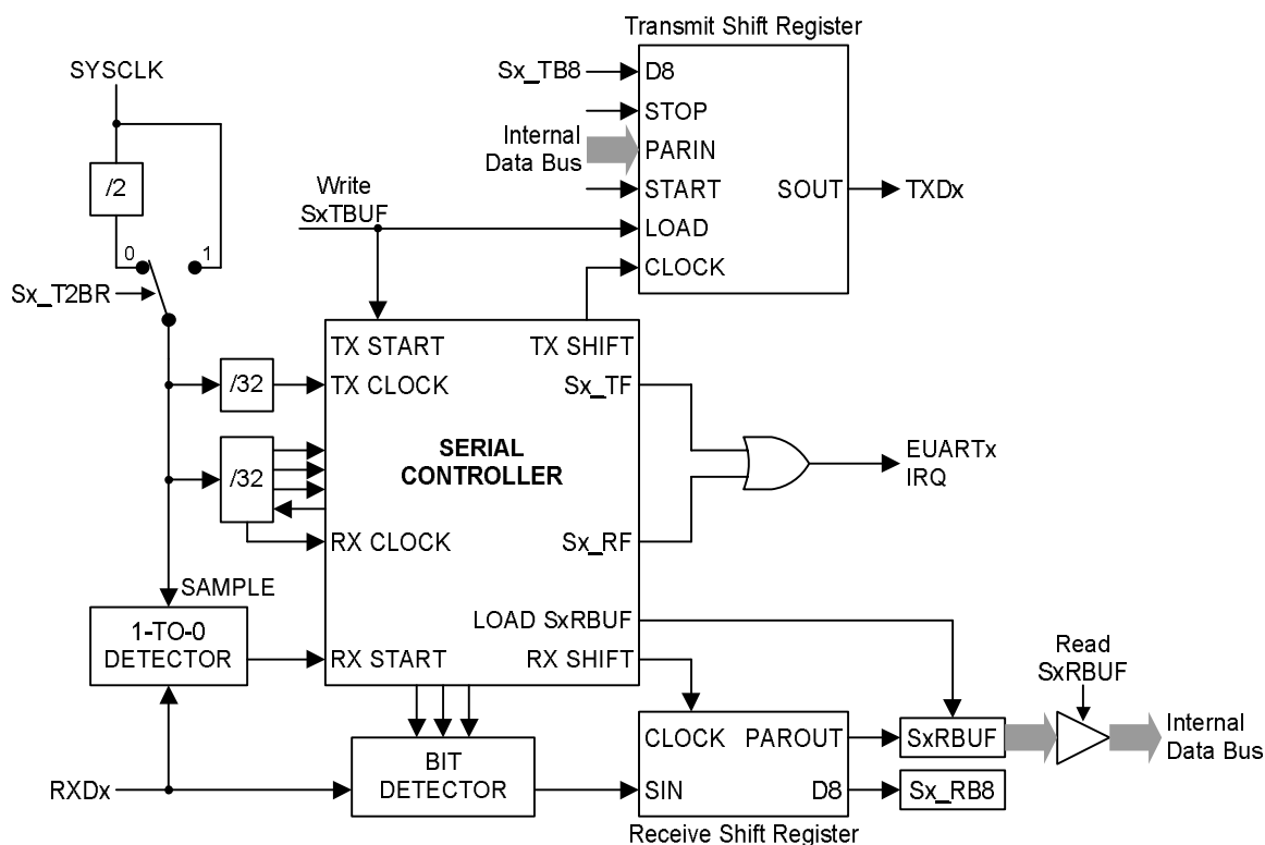
图 30. EUART 模式 2 结构框图
