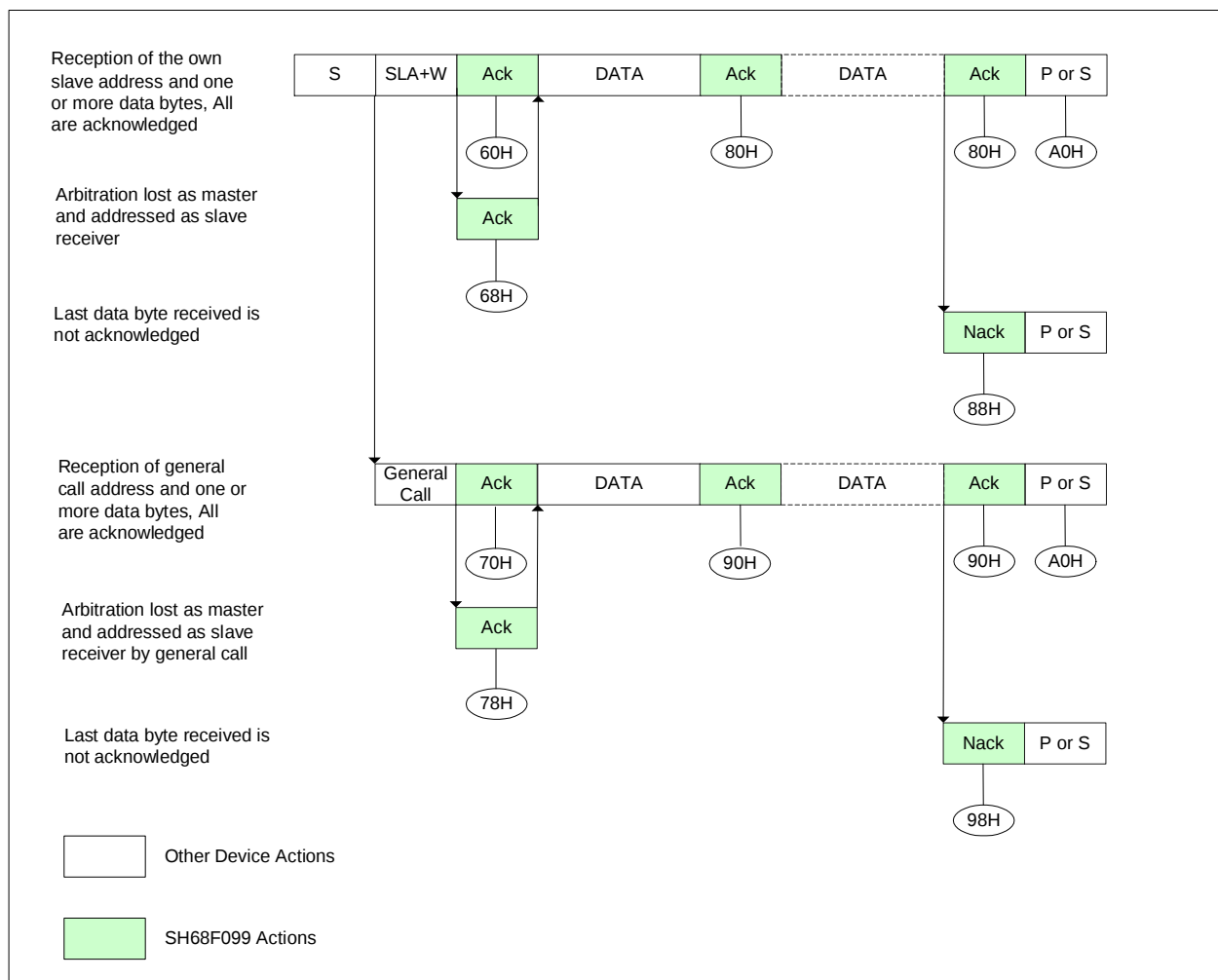
图 59. TWI 从机接收模式状态转换图
