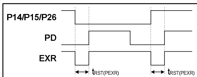
图 14. 关机模式端口复位 (PEXR) 时序图
