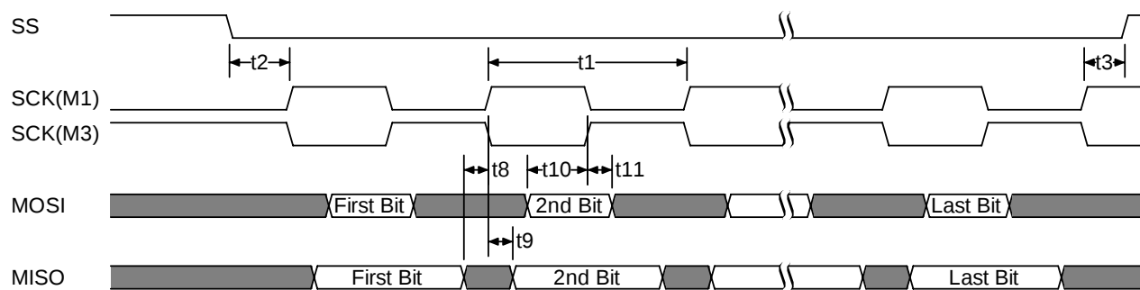
图 48. SPI Slave Mode 1、3 时序图
