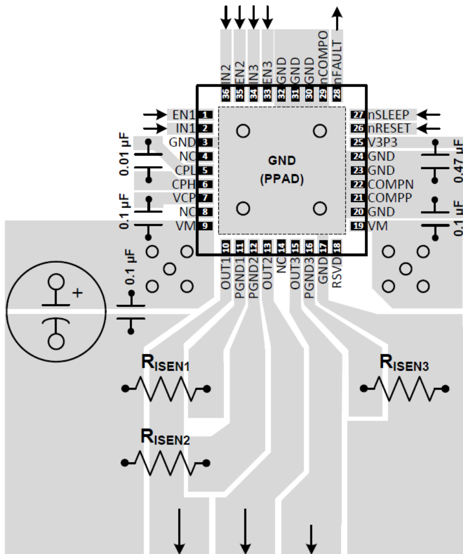
QFN36 PCB 布局参考
