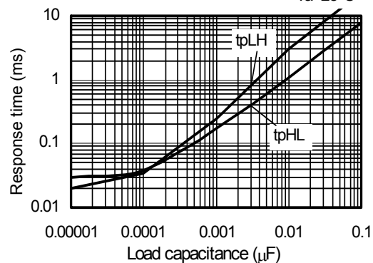
S-80960CN T_a=25^\circ\text{C}
