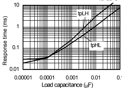
S-80960CN T_a=25^\circ\text{C}
