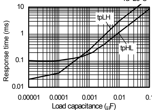
S-80960CN T_a=25^\circ\text{C}
