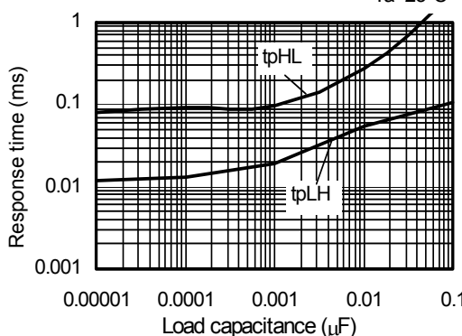
S-80960CL T_a=25^\circ\text{C}
