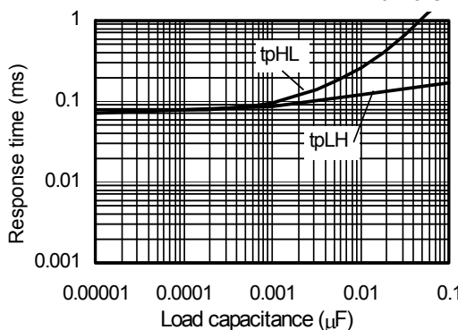
S-80960CL T_a=25^\circ\text{C}
