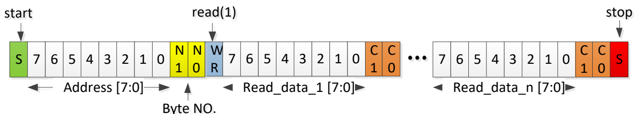
图 5.5 OWI 读操作
