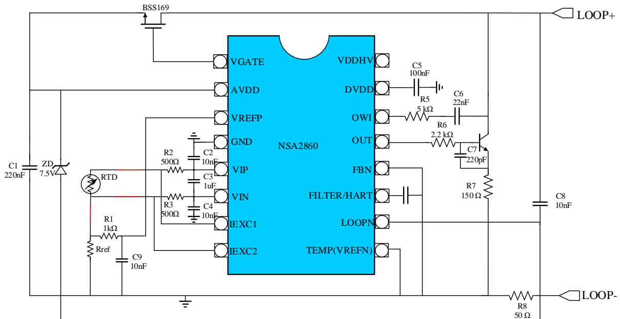
图 7.7 RTD 温度变送器
