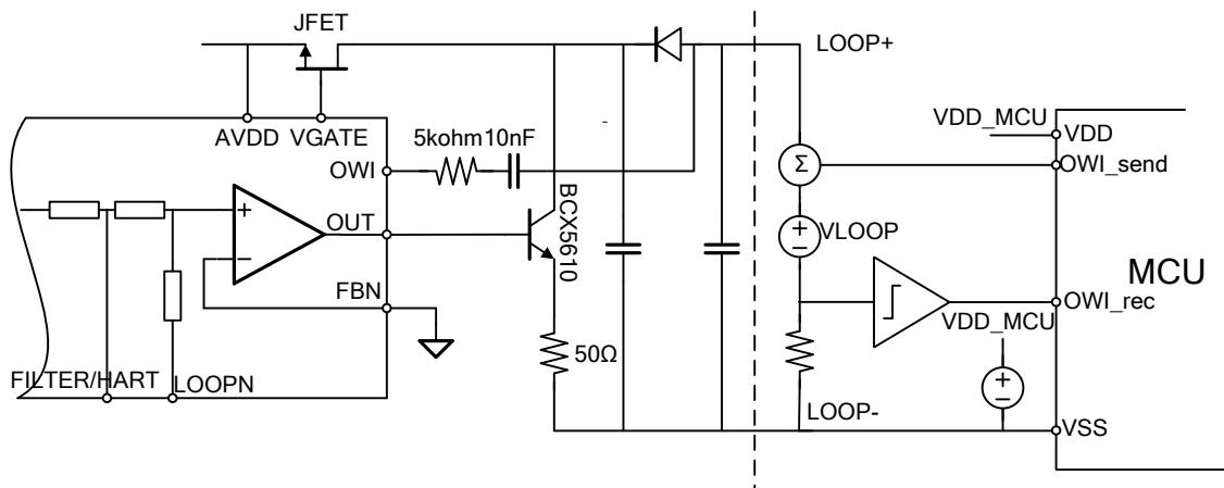
图 5.7 4~20mA 电流输出模式下双引脚 OWI 通讯典型连接图
