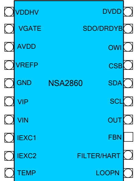
图 6.2 TSSOP-20 封装引脚分布
