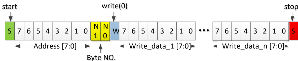
图 5.4 OWI 写操作
