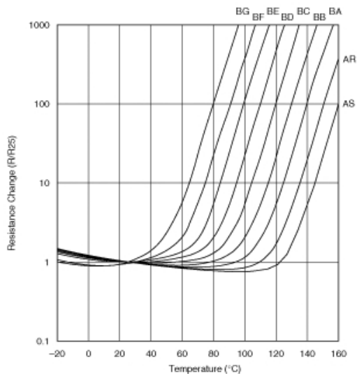
电阻-温度特性
