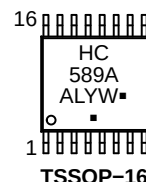
TSSOP-16
