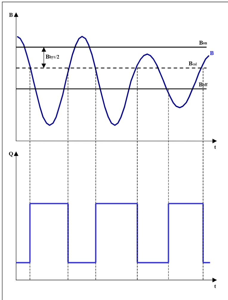
Fig. 2: Hidden hysteresis valid for programmed IC
