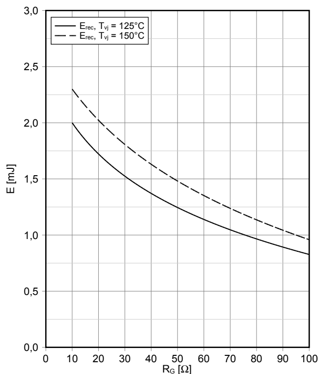
Schaltverluste Diode, Brems-Chopper (typisch) switching losses Diode, Brake-Chopper (typical) E_{rec} = f(R_G) I_F = 35\ \text{A} , V_{CE} = 600\ \text{V}
