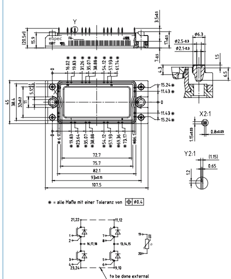
EconoPACK™2 B FourPACK M_E2e
