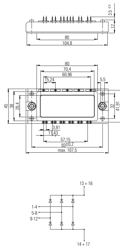
EconoBRIDGE™ Rectifier 2
