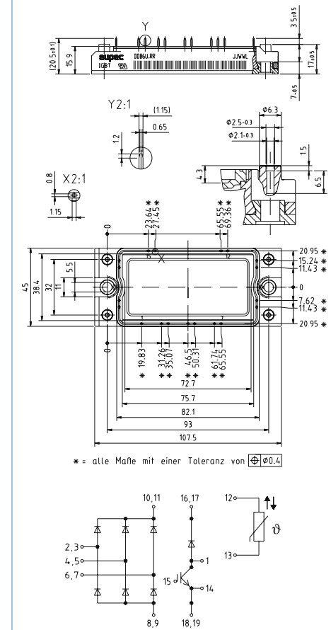
EconoBRIDGE™ Rectifier 2
