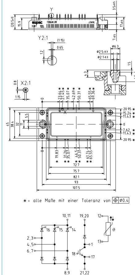
EconoBRIDGE™ Rectifier 2
