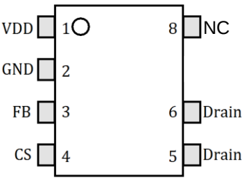
俯视图
