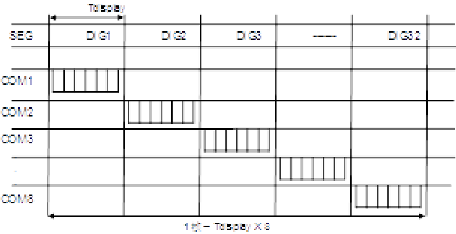
图 18-2-1-2 LED 驱动波形
