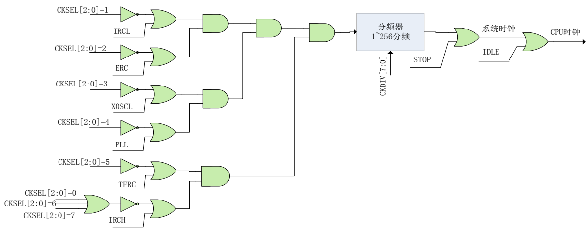
图 9-3-1-1 系统时钟结构图
