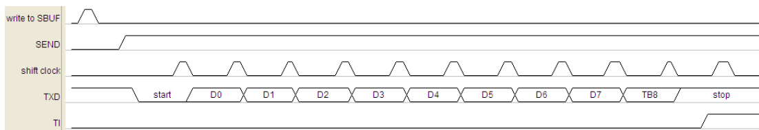
图 16-1-1-10 UART0 模式 2 发送数据波形
