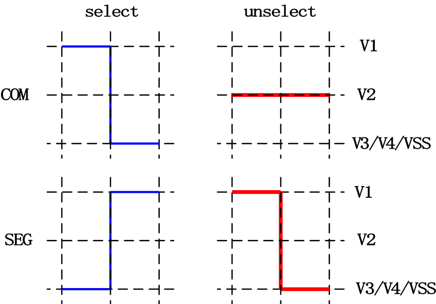
图 18-1-2-1 LCD 偏压比 1/2 信号
