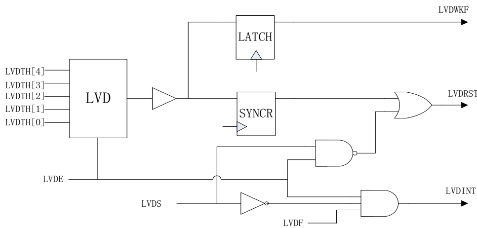
图 22-1-1 LVD 模块示意图
