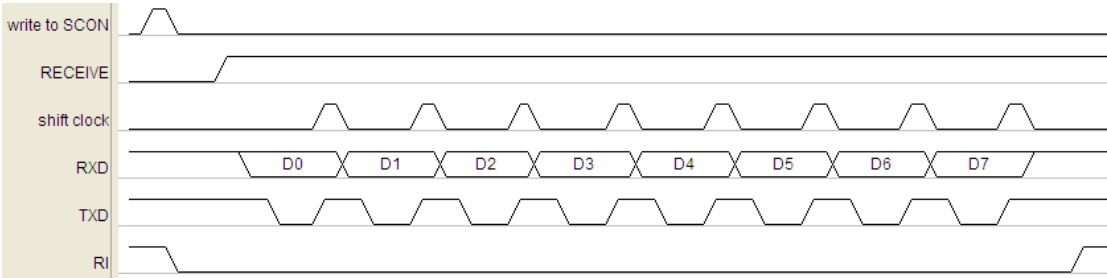
图 16-1-1-5 串口 0 模式 0 接收数据波形
