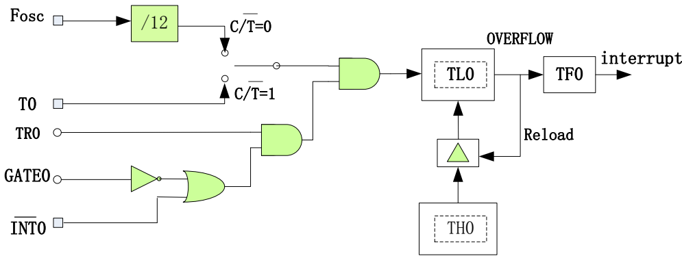
图 12-1-1-2 定时器 0 的模式 2
