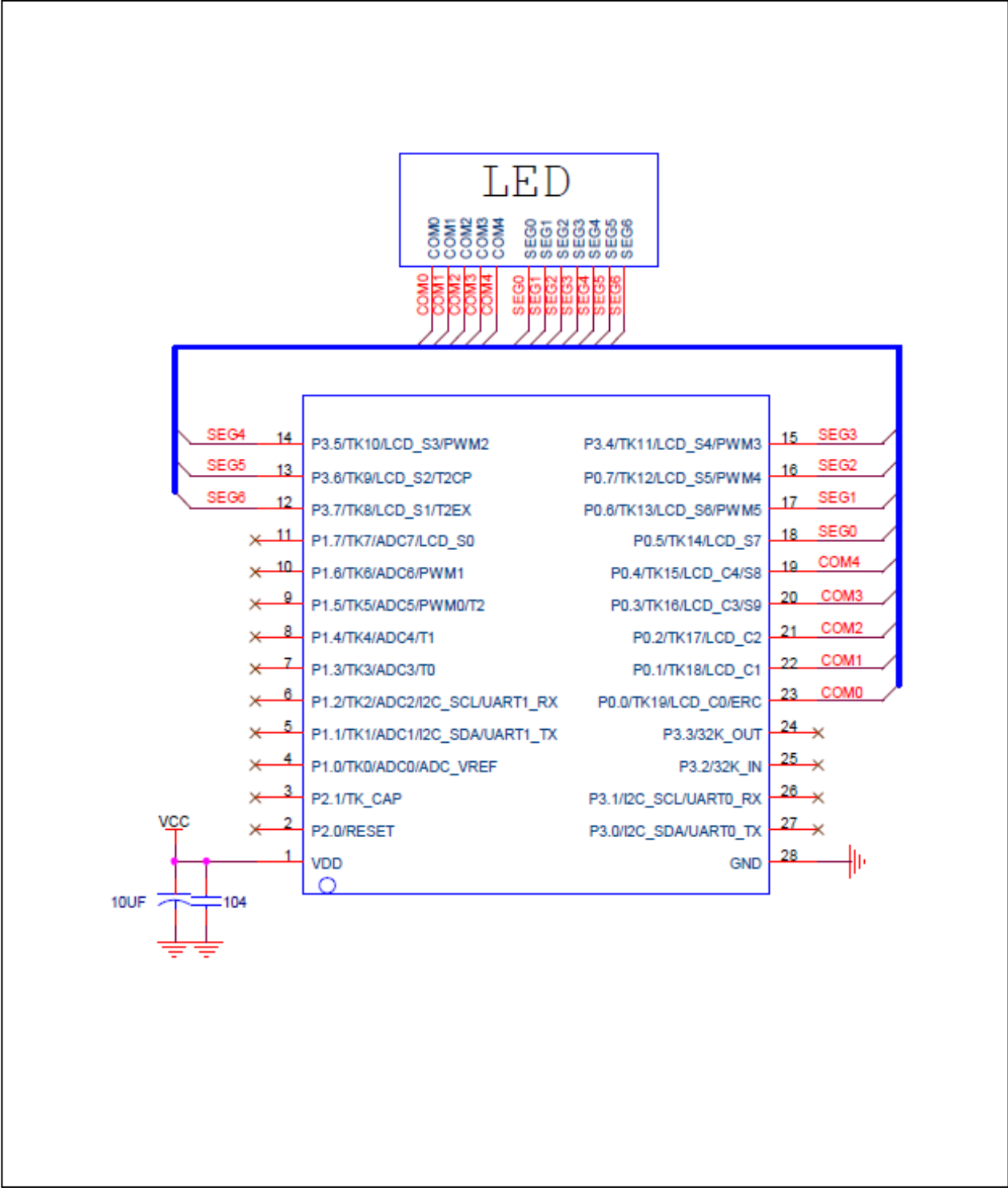
参考电路（一）
