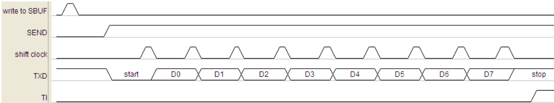
图 16-1-1-7 UART0 模式 1 发送数据波形
