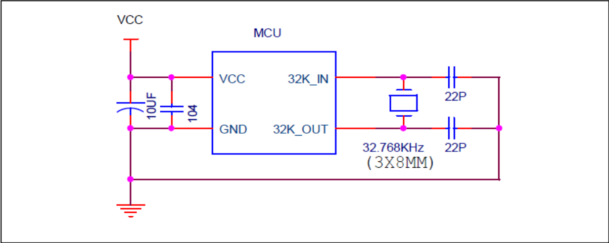
图 14-1-2 XOSC 典型电路图
