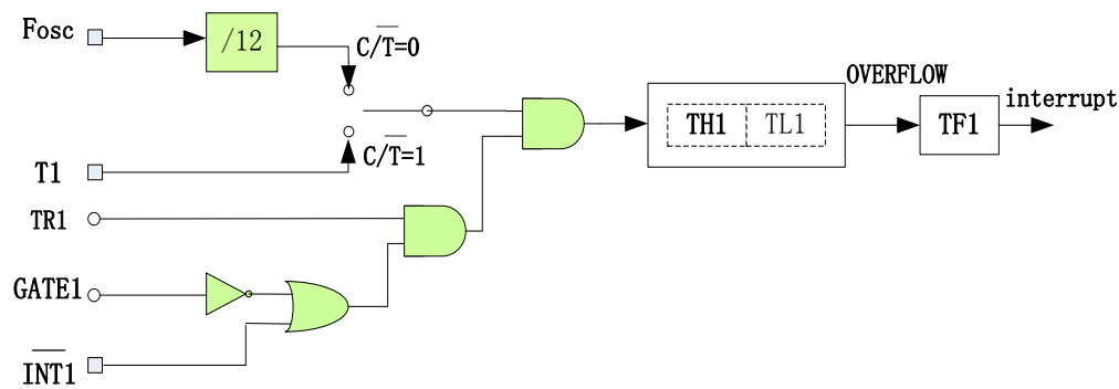
图 12-2-1-1 定时器 1 的模式 1
