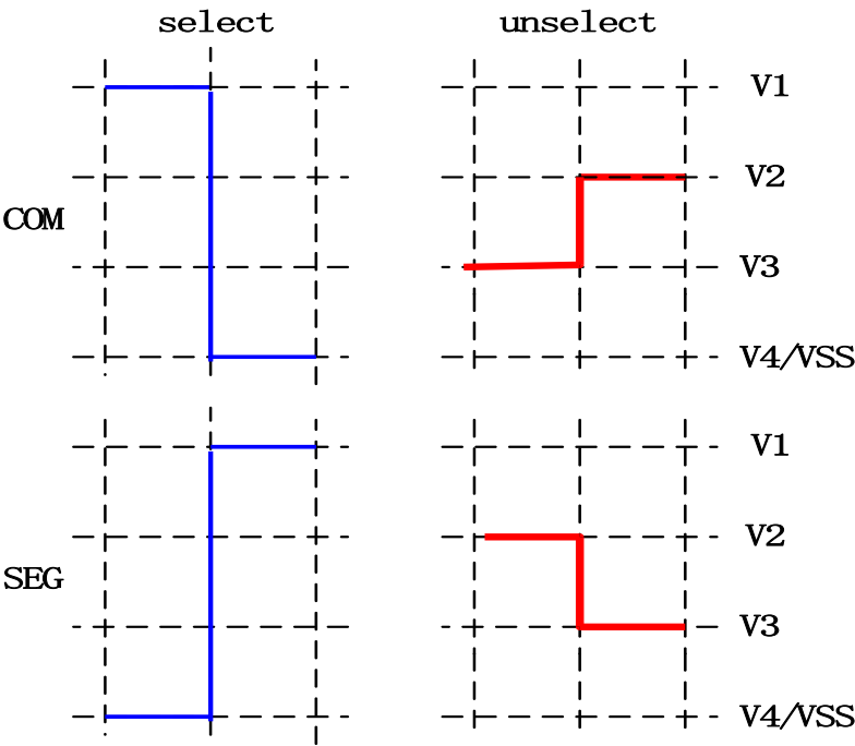
图 18-1-2-2 LCD 偏压比 1/3 信号
