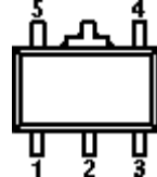
SOT-89-5L
