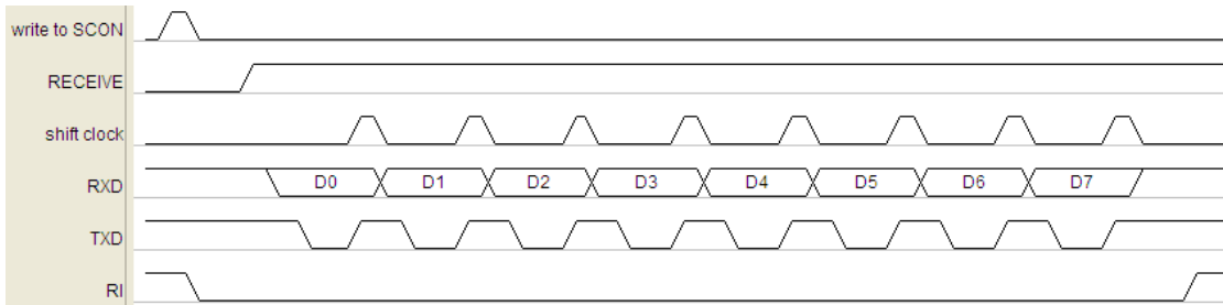
图 17-1-1-3 串口 0 模式 0 接收数据波形
