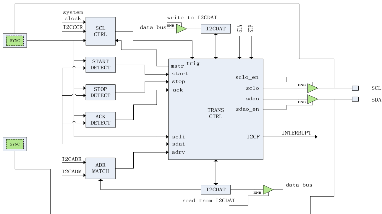
图 19-3-2 I²C 模块原理示意图
