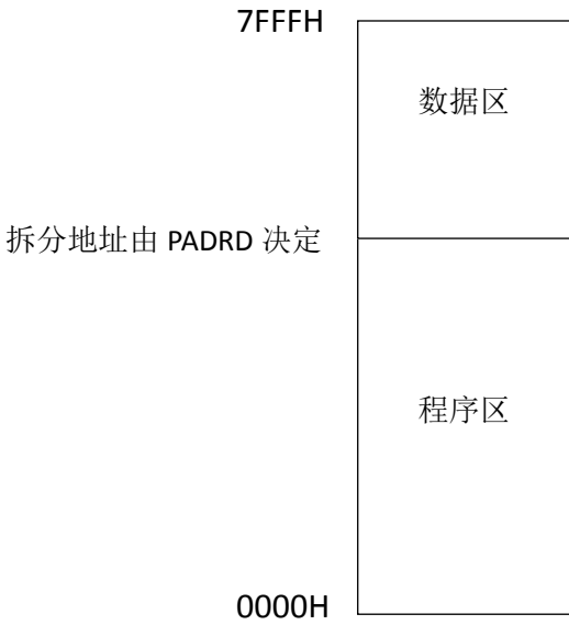
图 7-3-4 32K Flash 存储器结构
