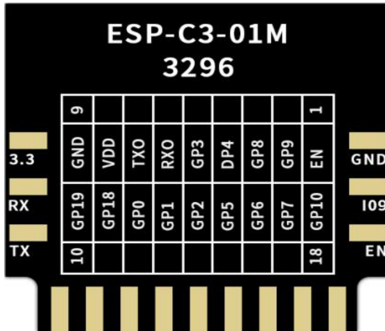
ESP-C3-01M 管脚示意图
