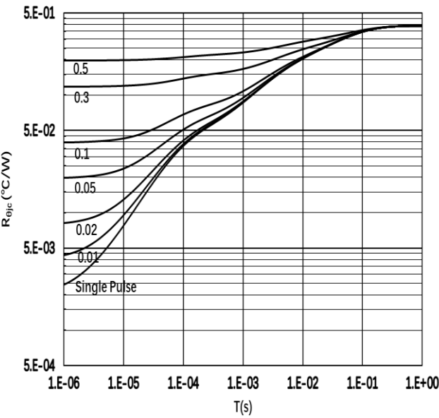
图 7 瞬态热阻抗
