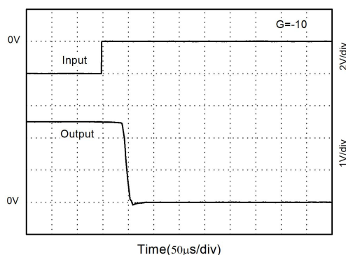
图6. 正过压恢复
