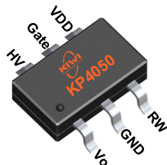
SOT23-6
