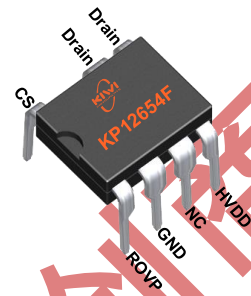
DIP-7
