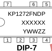
DIP-7
