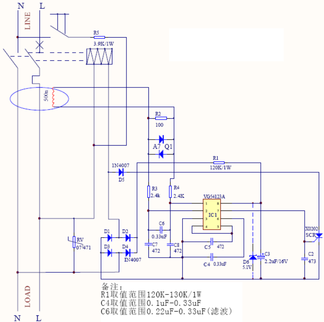
VG54123A 典型应用电路二
