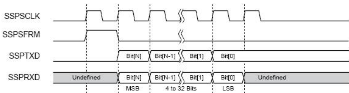
图 26: PCM 时序
