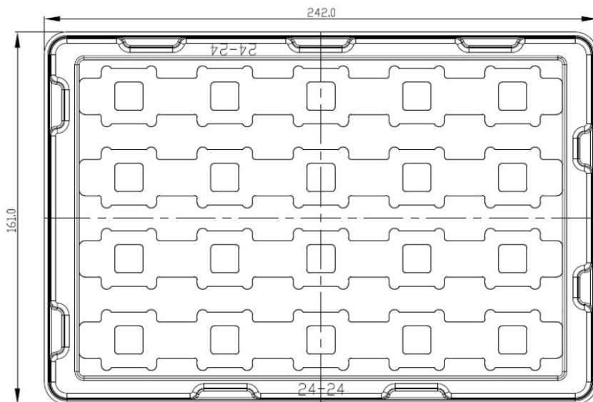
图 36: 托盘尺寸图
