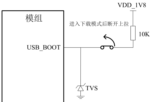
图 20: USB_BOOT 连接图
