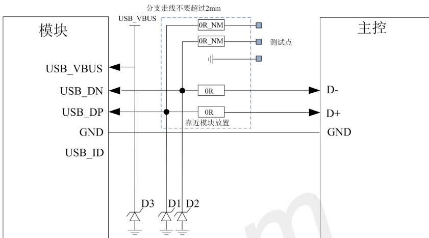
图 19：USB 连接图
