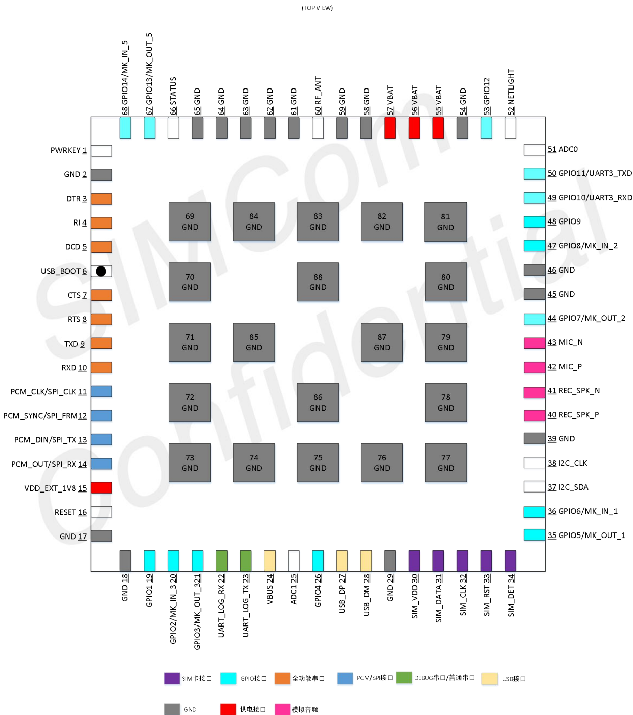
图 3：A7670C-LAAE/A7670C-LAAL/A7670C-LAAS 模块引脚图(正面视图)
