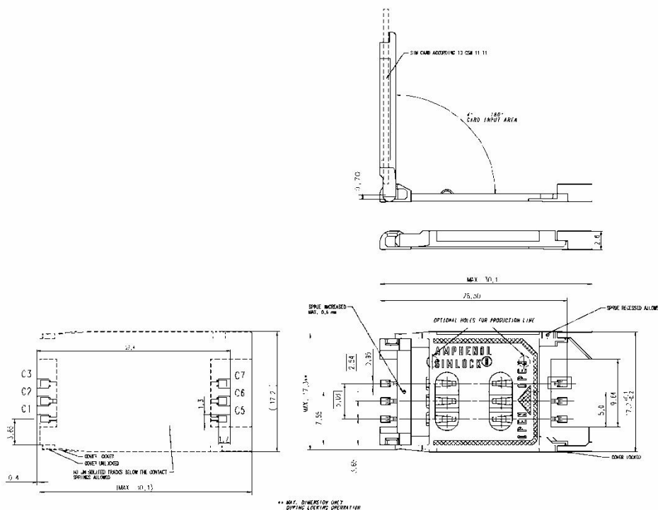
图 24: Amphenol C707 10M006 512 USIM 卡座尺寸图
