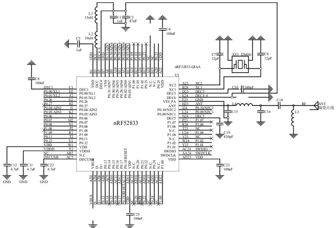
图 5-1 电路图
