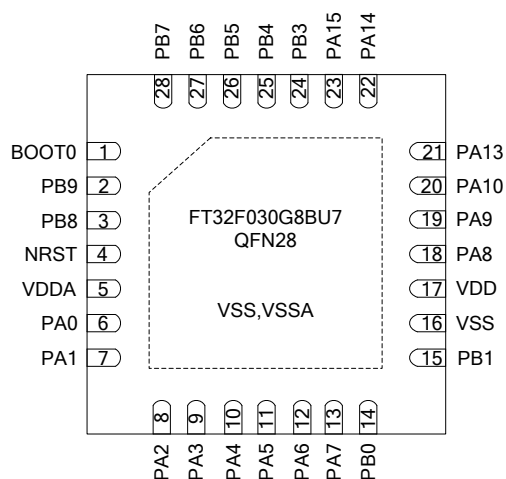
图 4.6 QFN28 引脚分配
