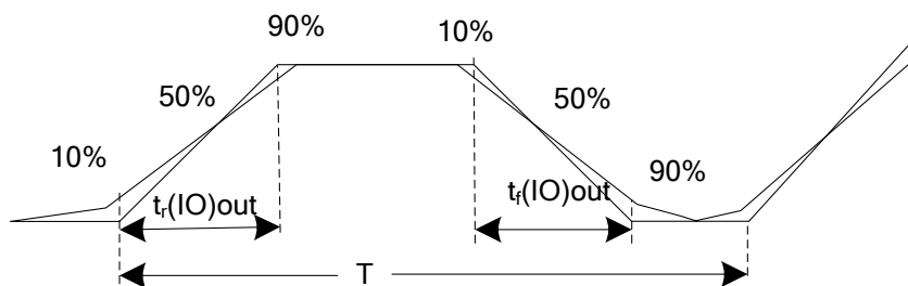
图6.10 I/O交流特性定义
