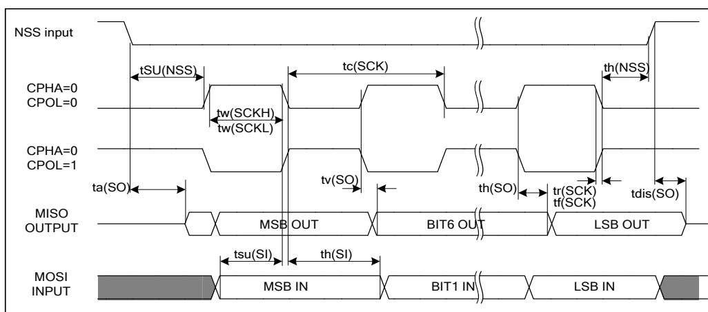
图 6.15. SPI 时序图-从模式并且 CPHA=1
