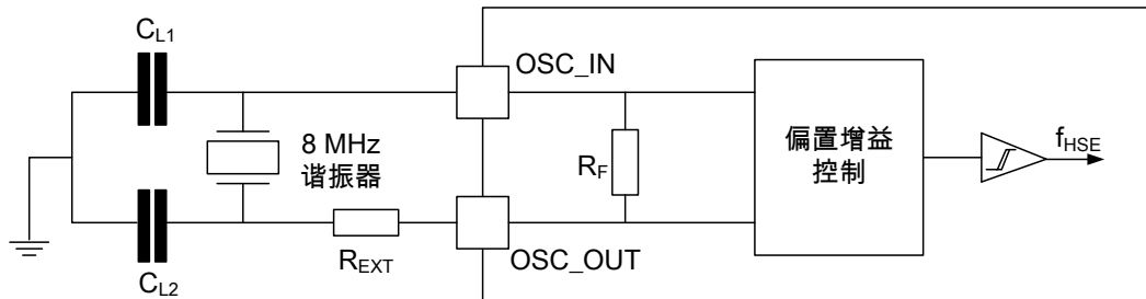
图 6.7 使用 8MHz 晶体的典型应用
