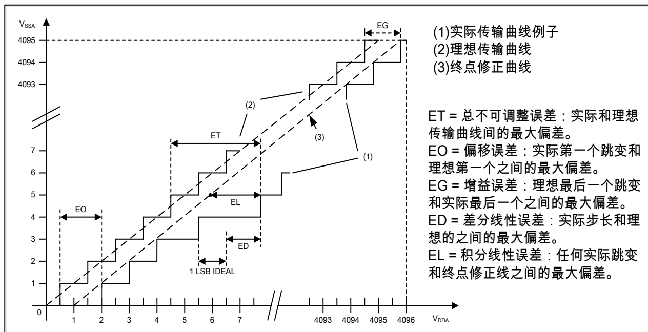
图 6.12 ADC 精度特性
