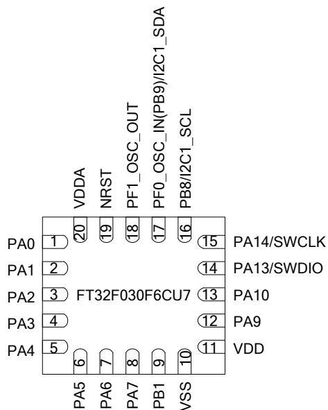
图 4.5 QFN20 引脚分配
