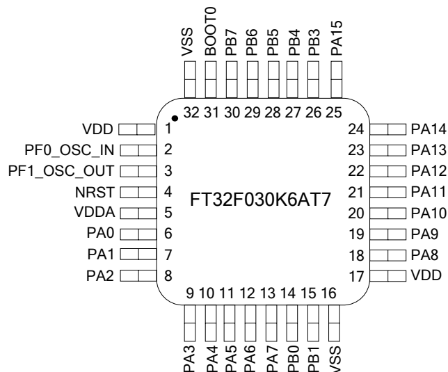
图 4.3 LQF32 引脚分配
