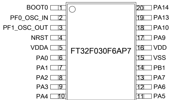
图 4.4 TSSOP20 引脚分配
