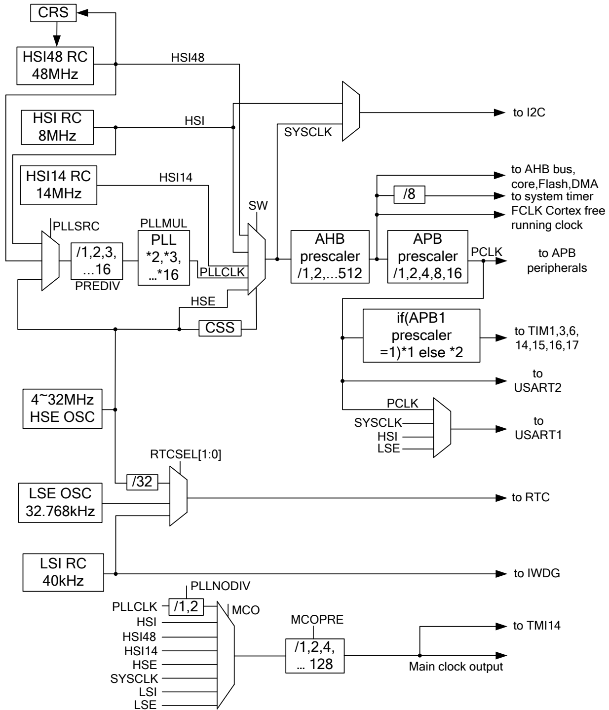
图 3.1 时钟框图
