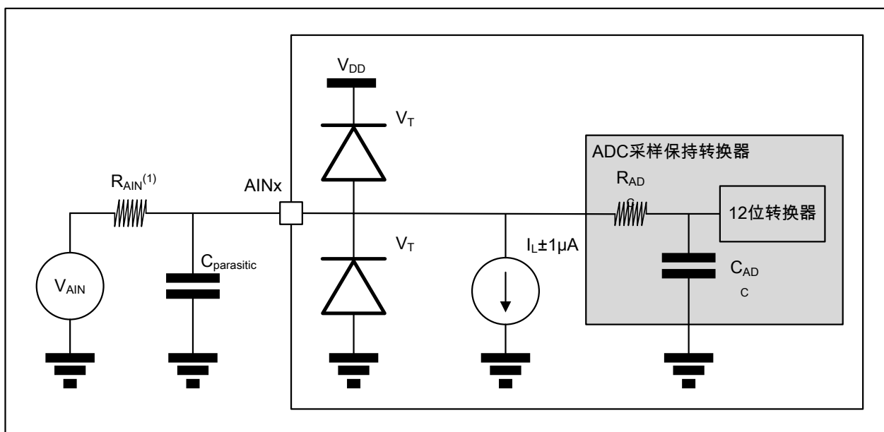
图 6.13 ADC 典型应用连接图
